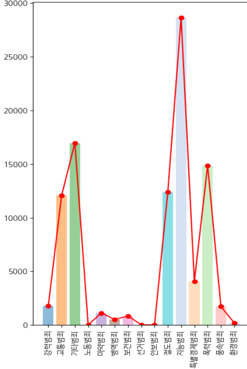
특별/광역시 범죄 건수(평균)
