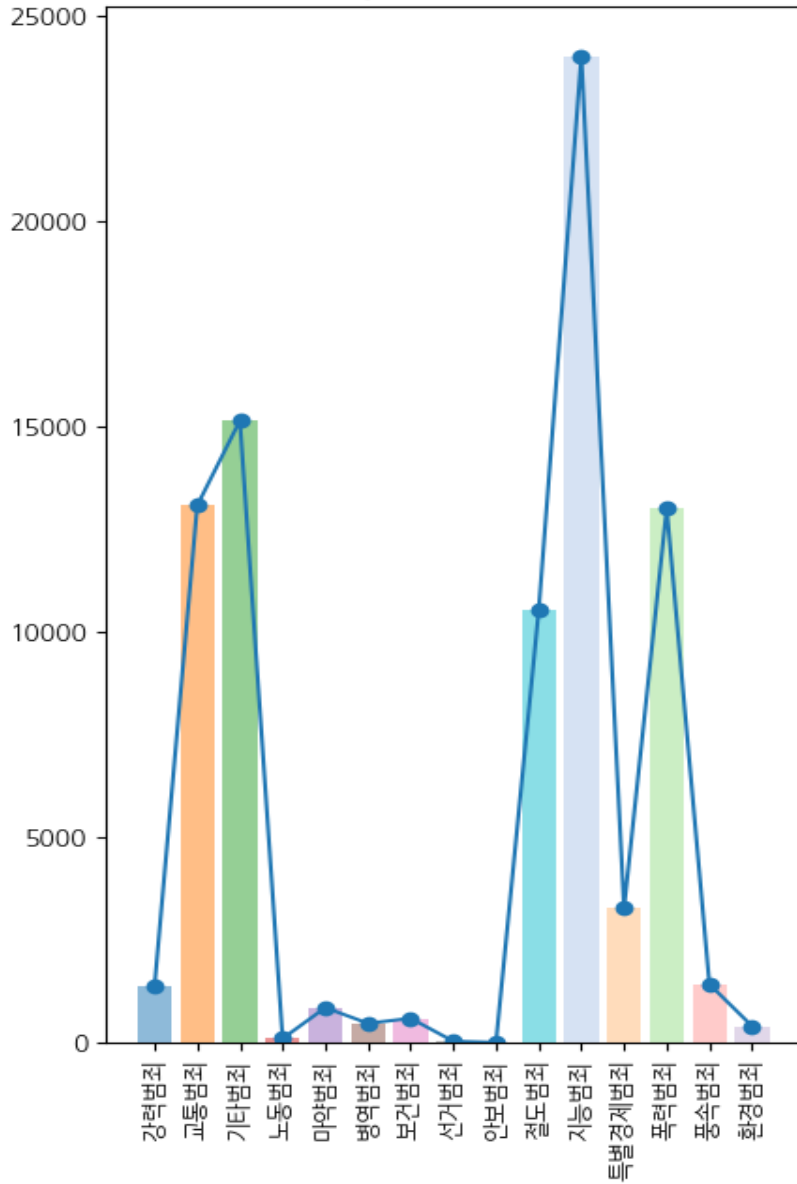
전국 범죄 건수(평균)
