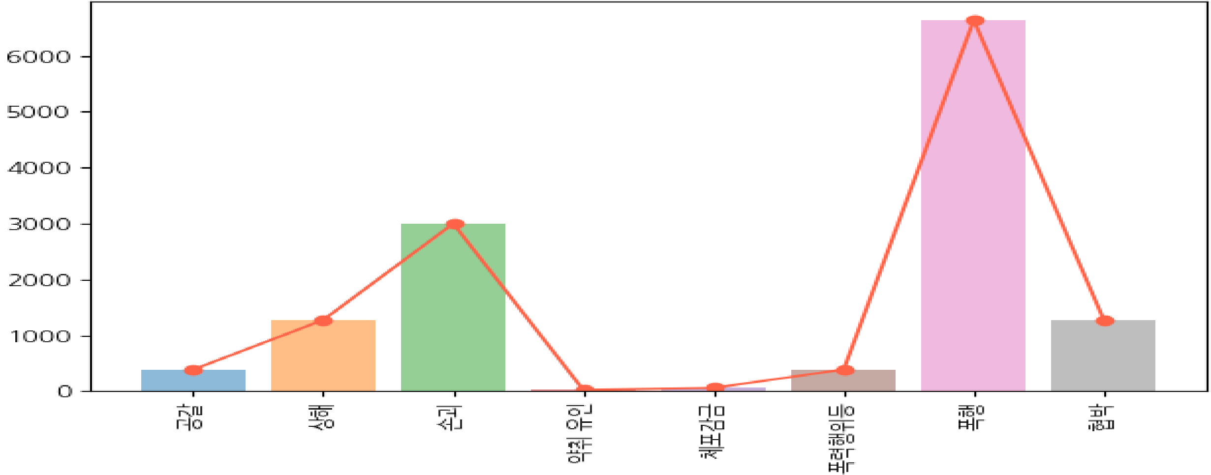
폭력범죄 유형별 건수평균
