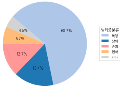
식당 및 유흥 시설
