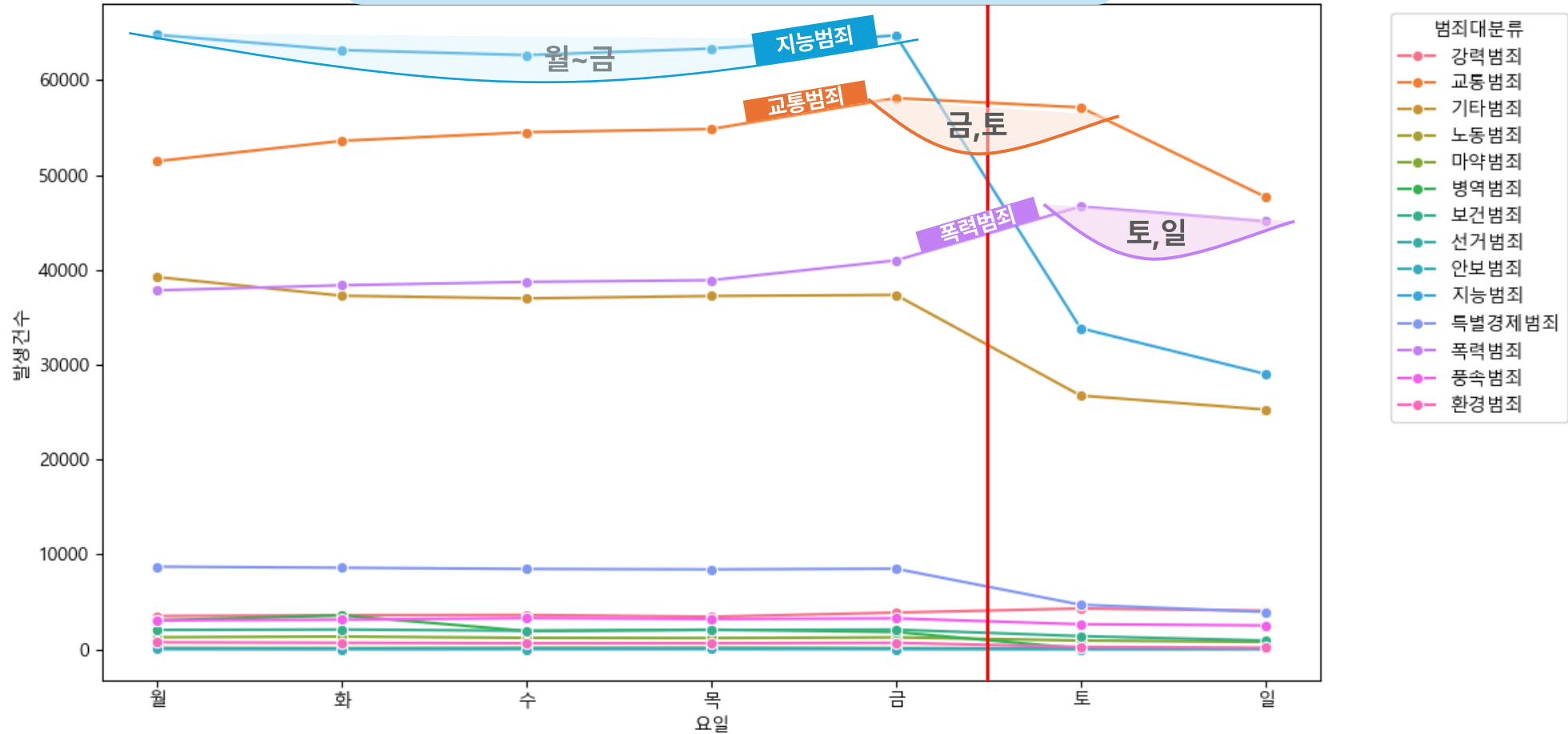
범죄대분류별 요일별 발생 패턴
