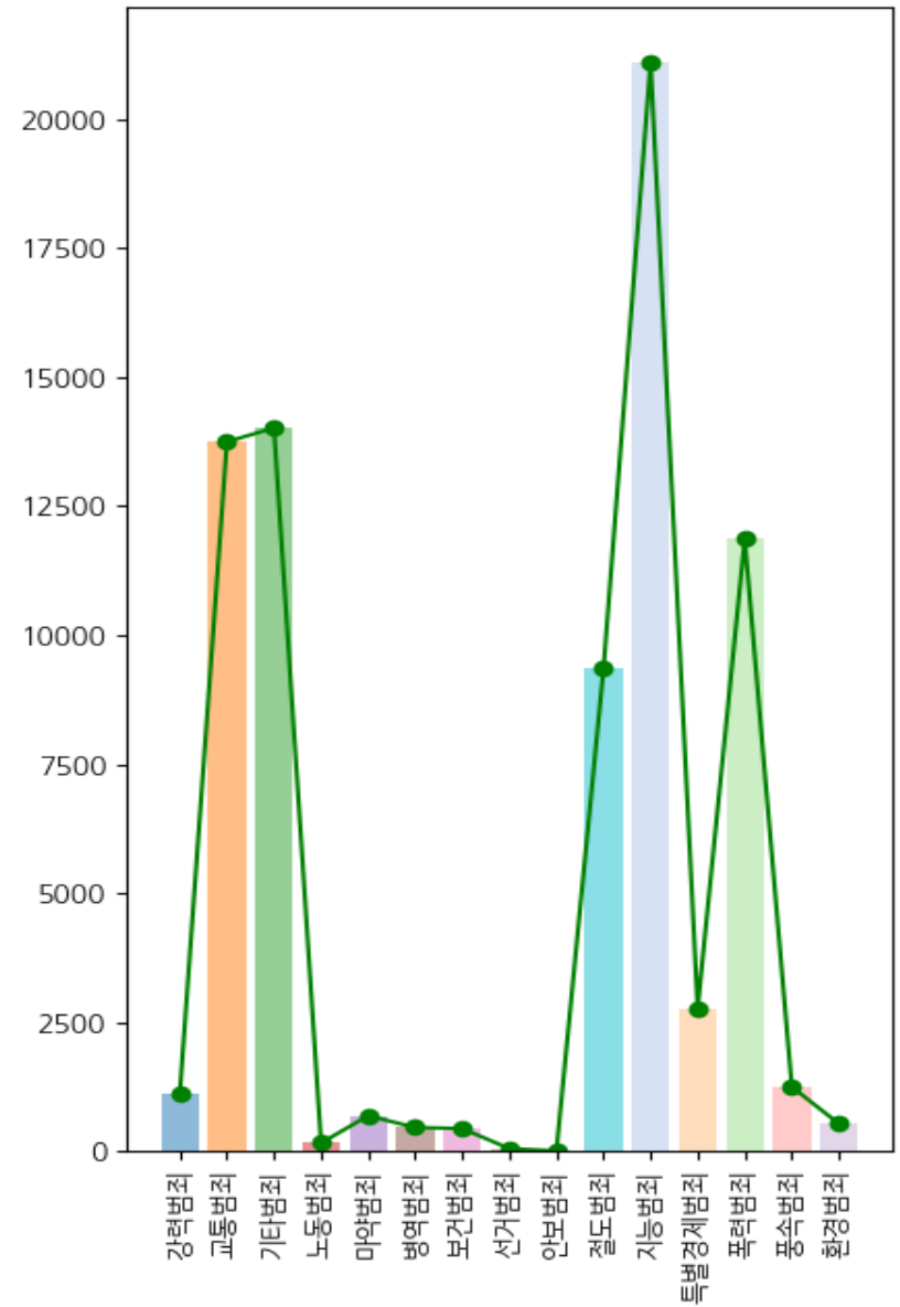
도/군/구 범죄 건수(평균)
