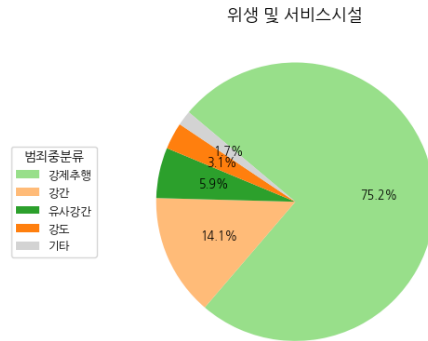
강력 범죄율 상위 8개 장소 범죄중분류
