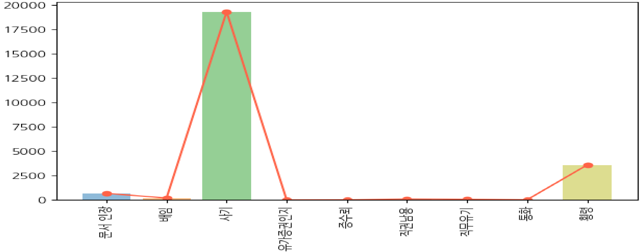
지능범죄 유형별 건수평균
