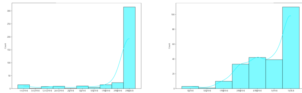
증수뢰 인지/검거기간 분포
