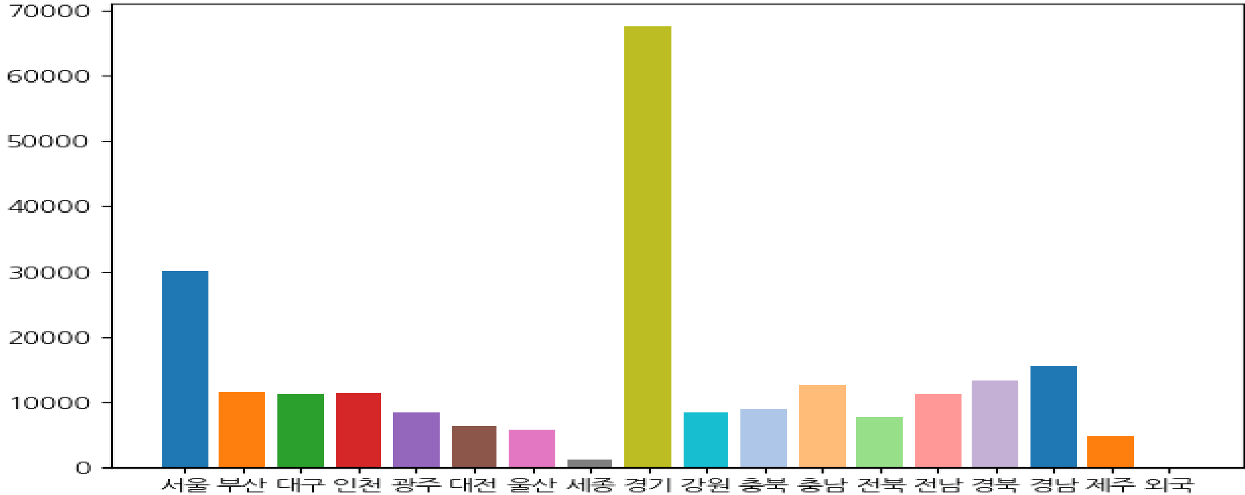
교통범죄 전체 건수
