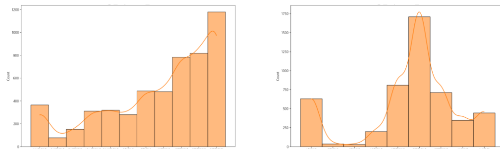
강간 인지/검거기간 분포
