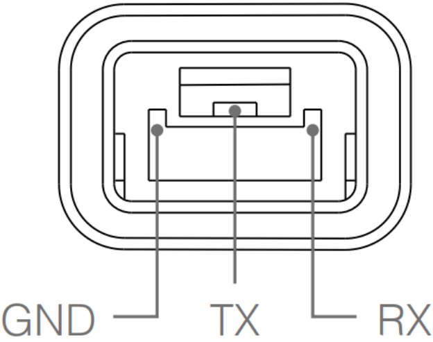
图 8-2 发送端 uart 串口线序
