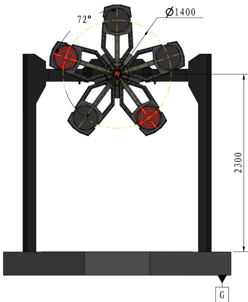
图 4-29 能量机关示意图
