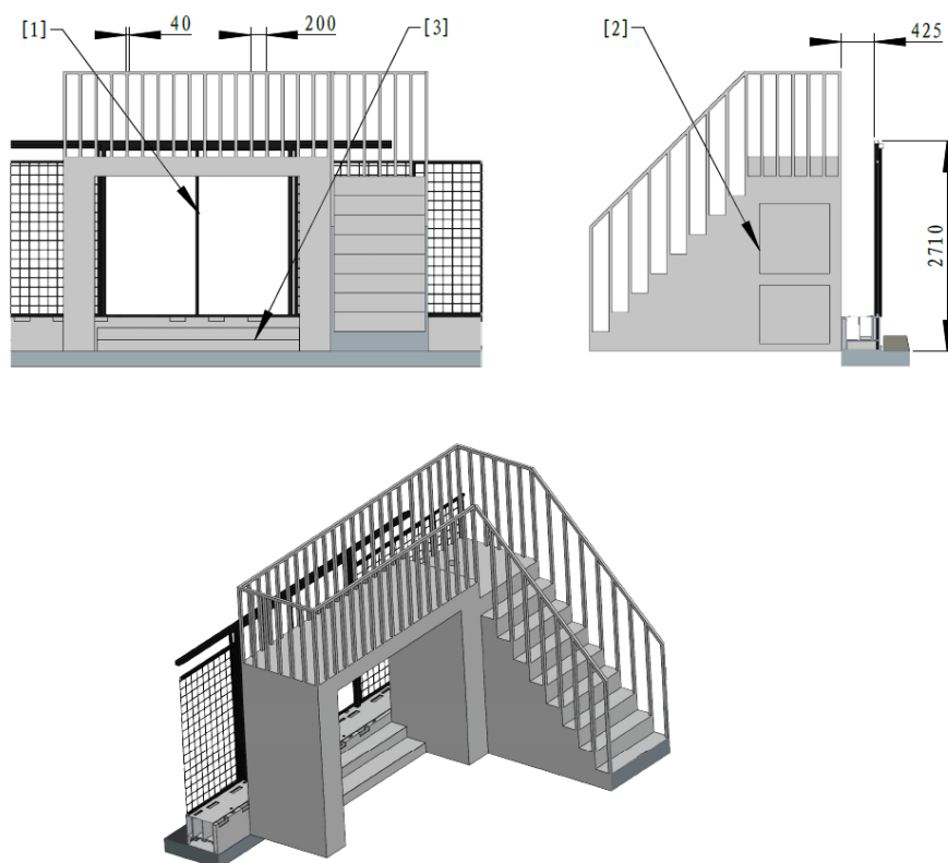
[1] 战场出入口 [2] 雷达基座 [3] 出入口台阶
