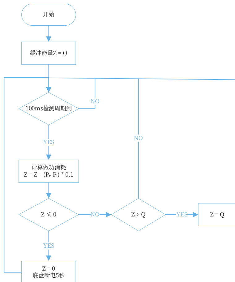
图 5-3 机器人底盘功率检测及超限惩罚机制
