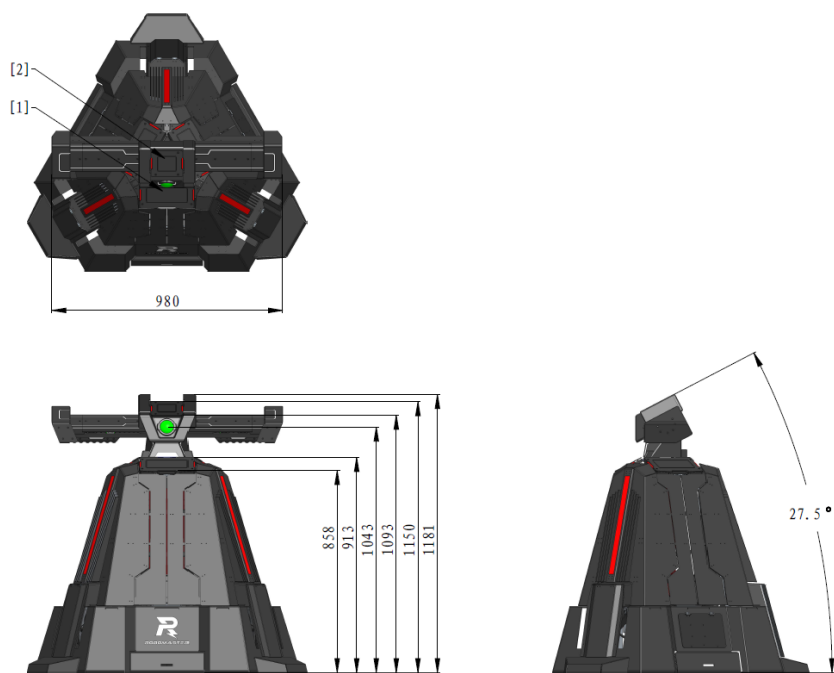
[1] 大装甲模块 [2] 飞镖检测模块
