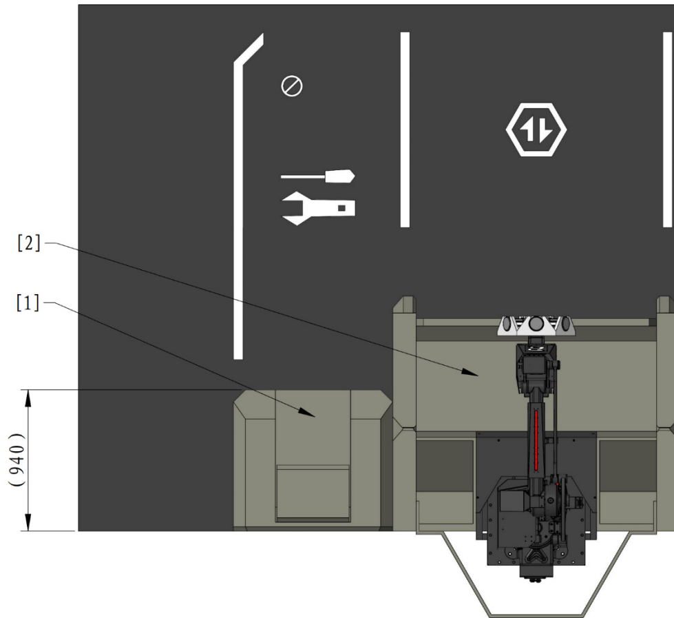
[1] 无线充电装置放置区 [2] 资源区
