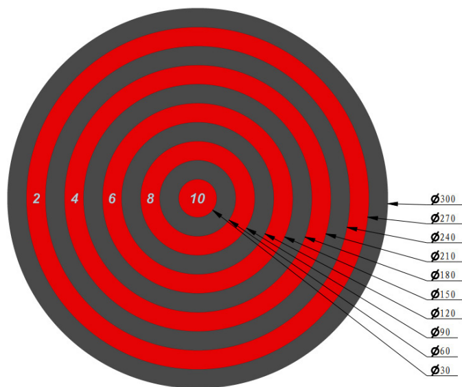
图 5-11 能量机关击打区域示意图
