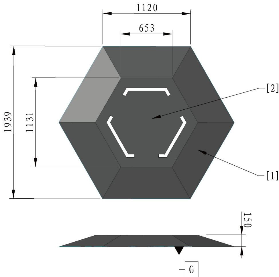
[1] 20°坡 [2] 堡垒增益点
