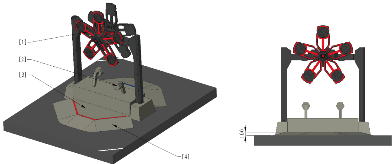
[1] 能量机关 [2] 科技核心 [3] 装配区 [4] 10°坡
