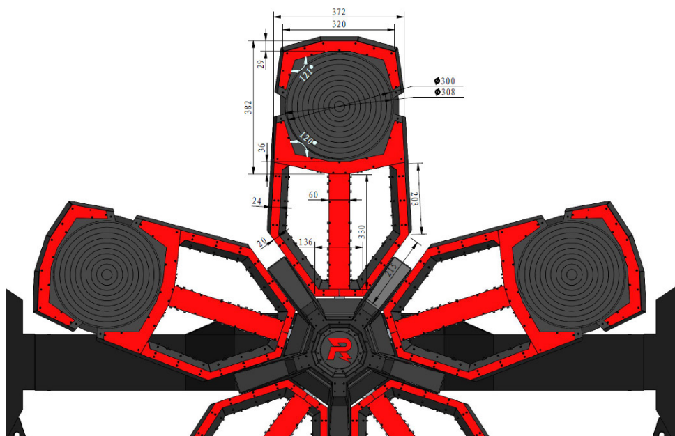
图 4-30 能量机关灯臂尺寸示意图
