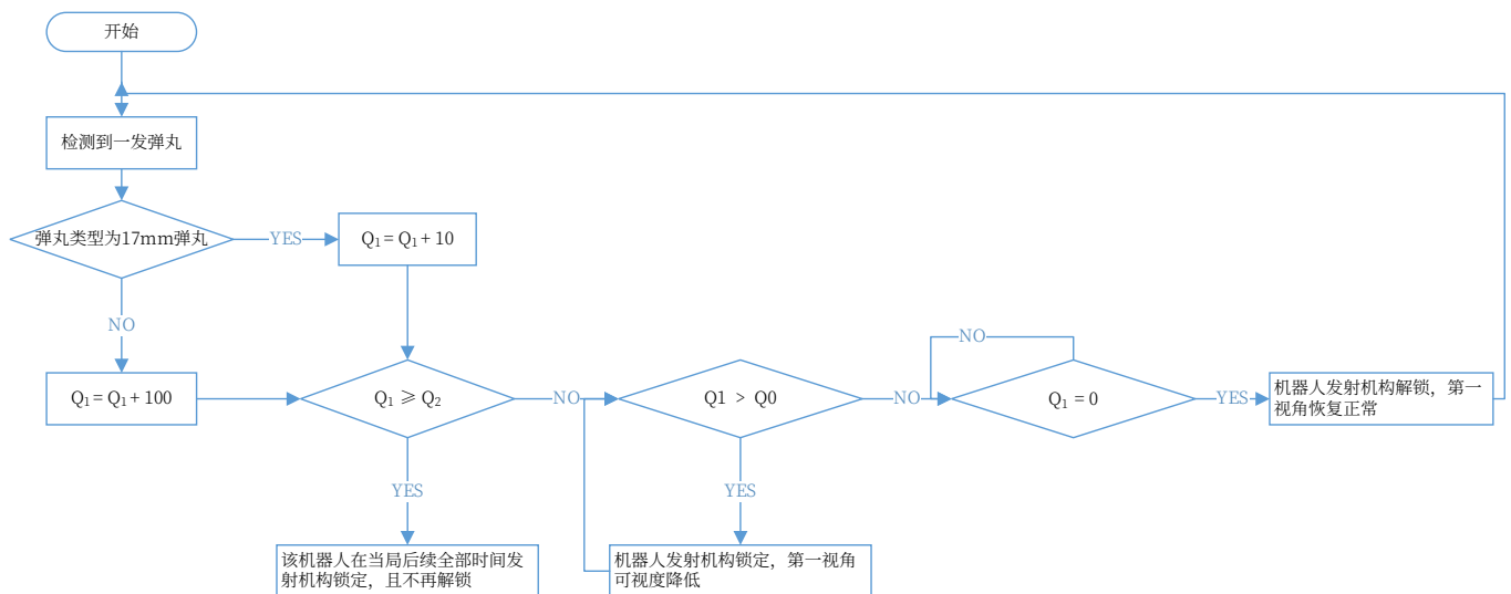
图 5-1 射击热量超限惩罚机制
