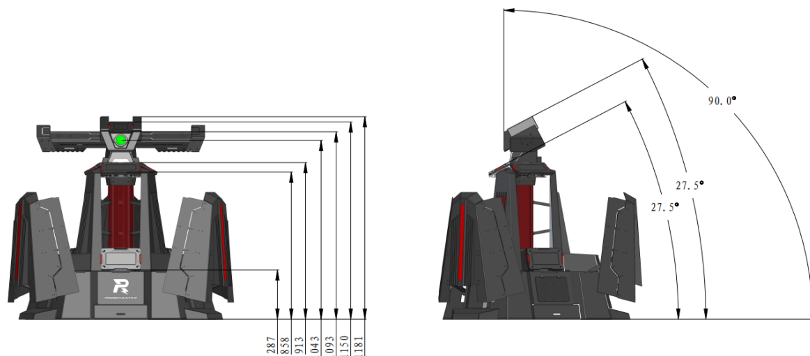
图 4-11 基地护甲展开形态尺寸图
