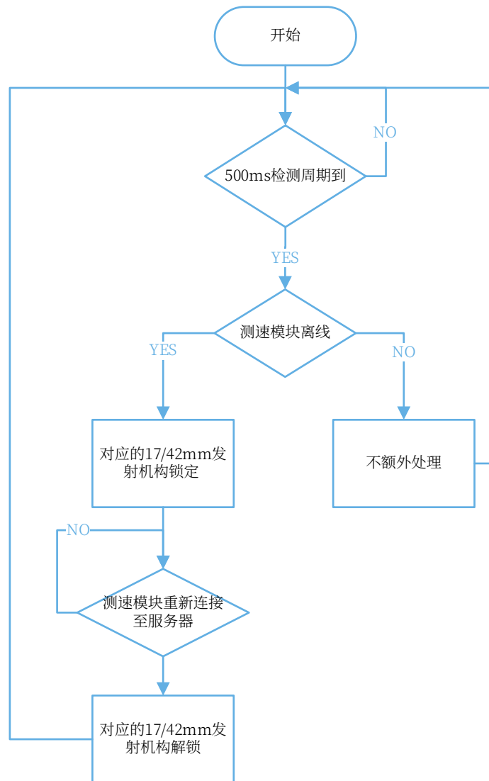
图 5-5 测速模块离线的断电机制
