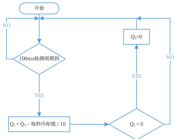
图 5-2 射击热量冷却机制
