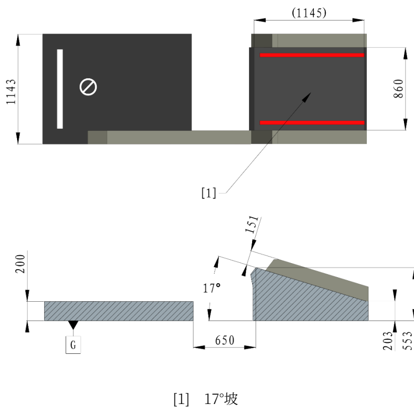
图 4-36 飞坡示意图
