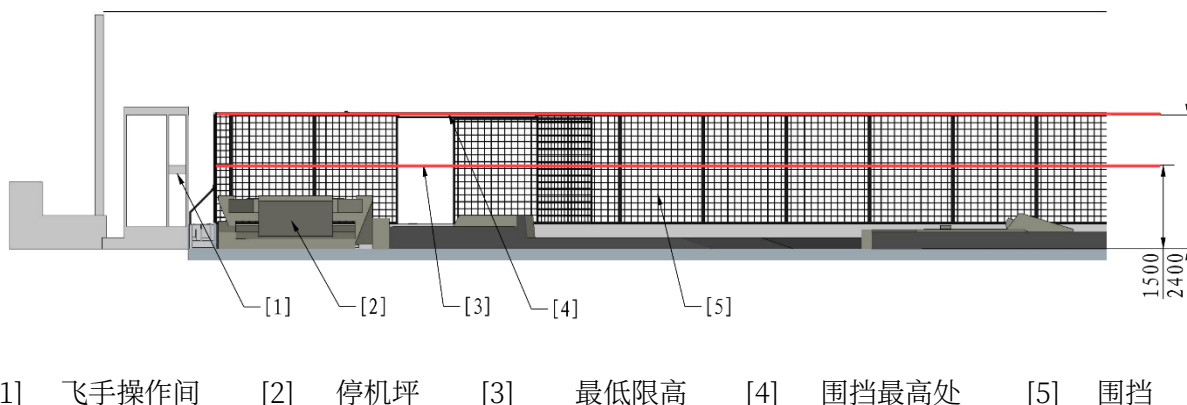
图 7-1 飞行高度限制示意图
