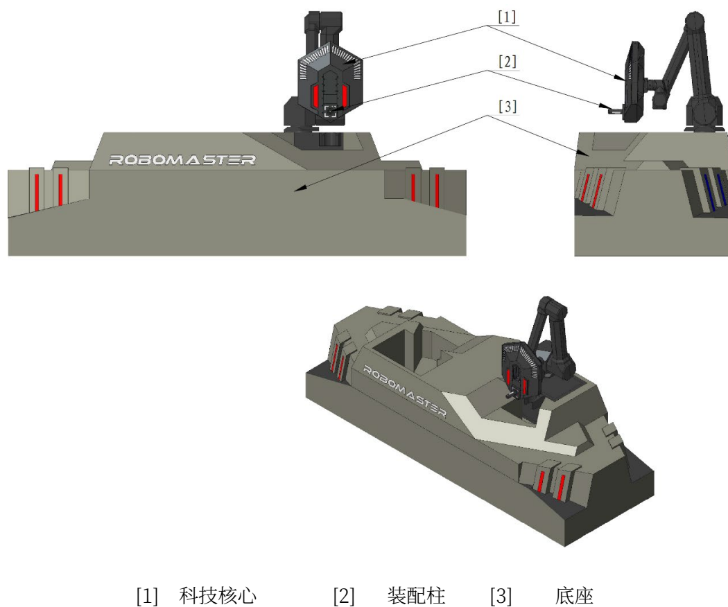
图 5-6 科技核心示意图
