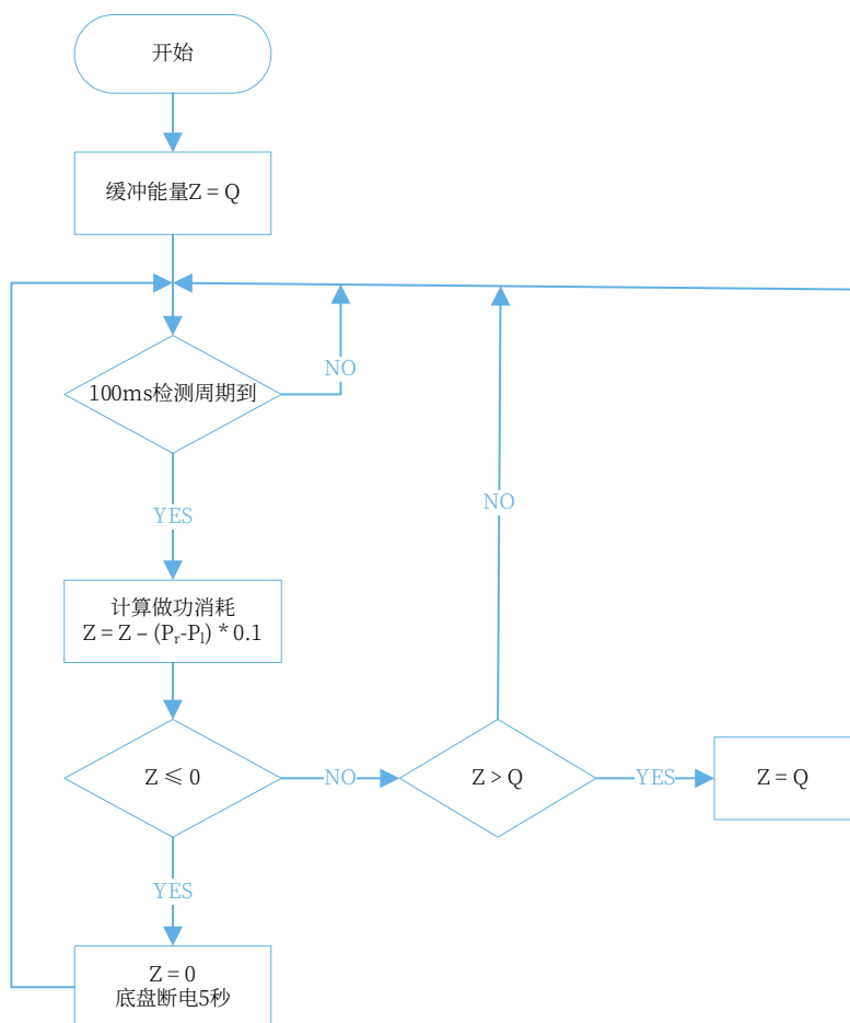
图 5-2 机器人底盘功率检测及超限惩罚机制
