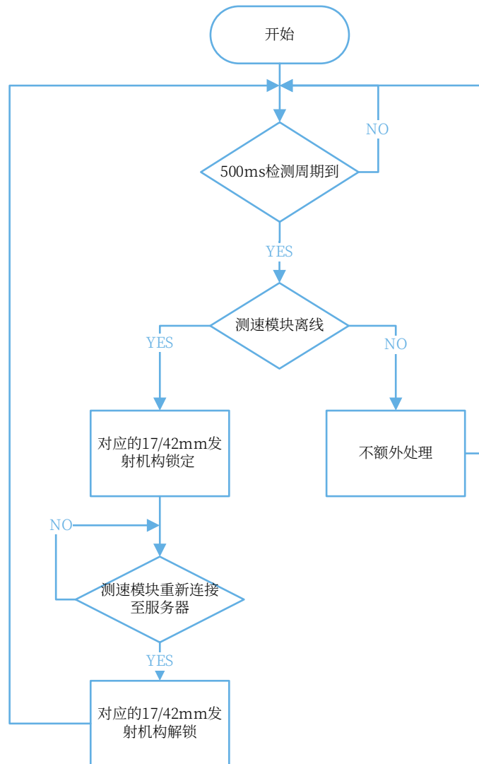
图 5-4 测速模块离线的断电机制
