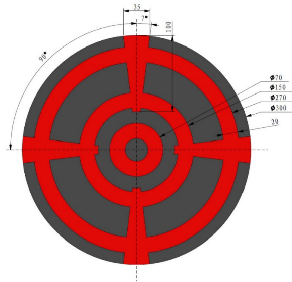
图 5-21 能量机关可激活标识示意图
