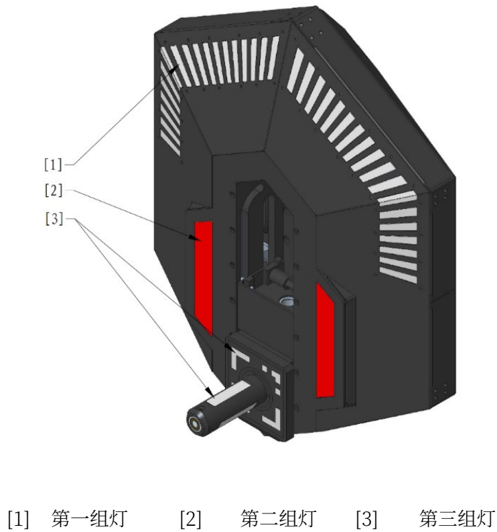
图 5-11 科技核心灯效示意图
