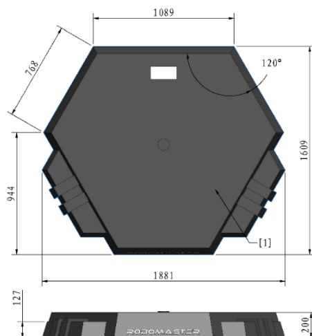
图 4-9 基地底座示意图
