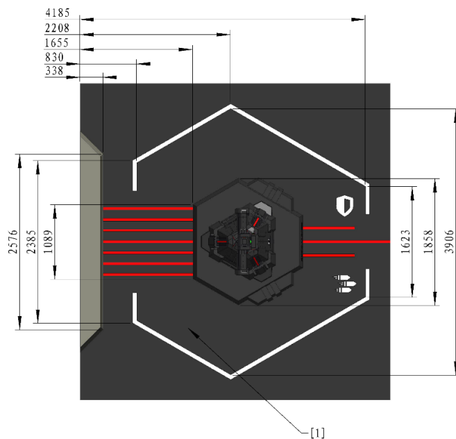
[1] 启动区
