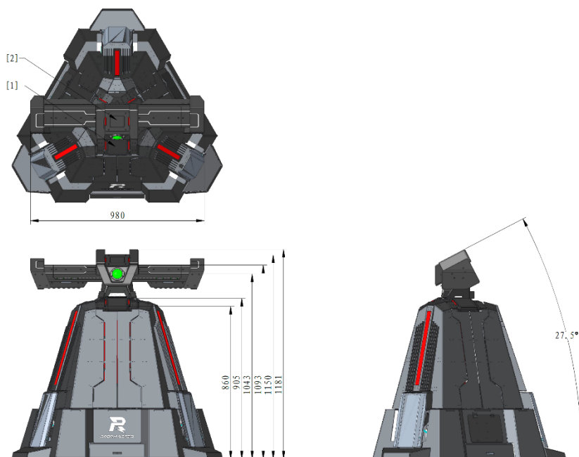
图 4-9 基地底座示意图
