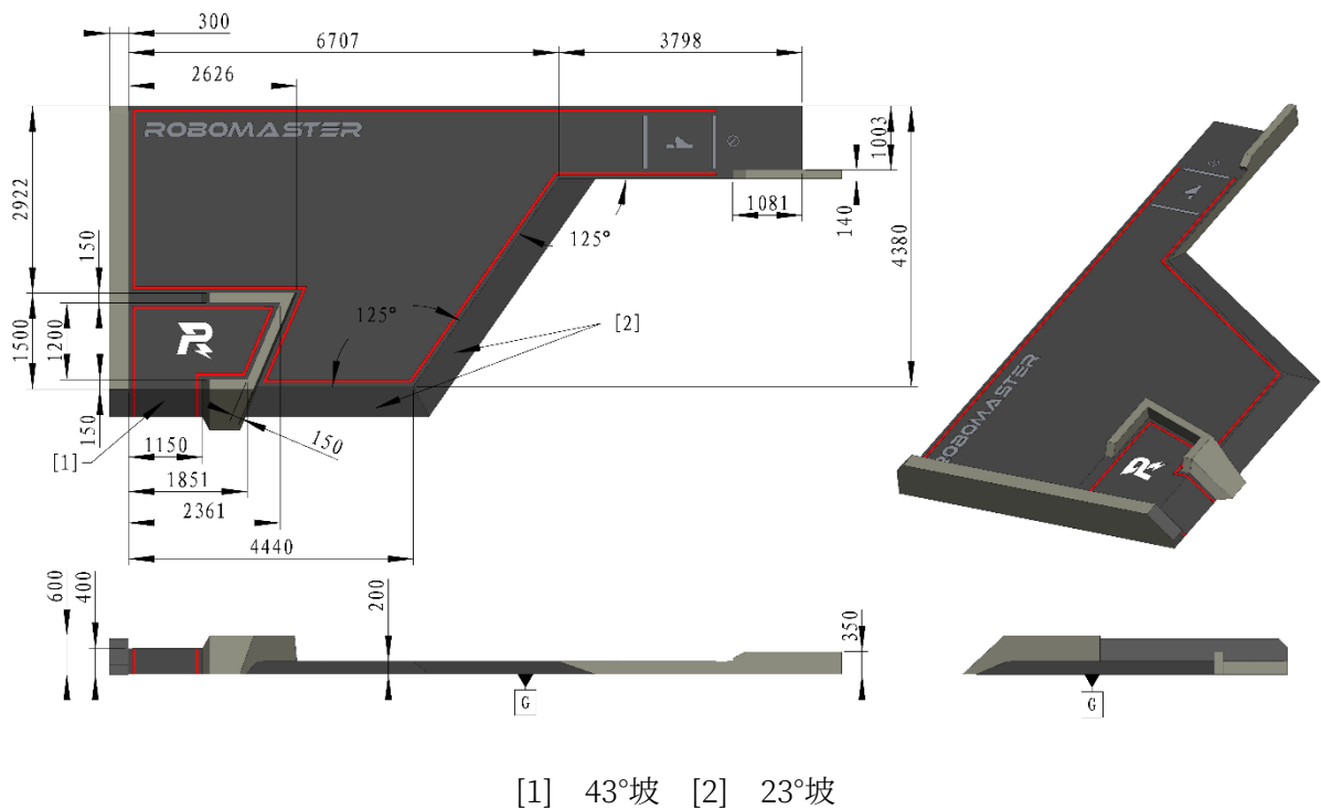
图 4-26 梯形高地示意图
