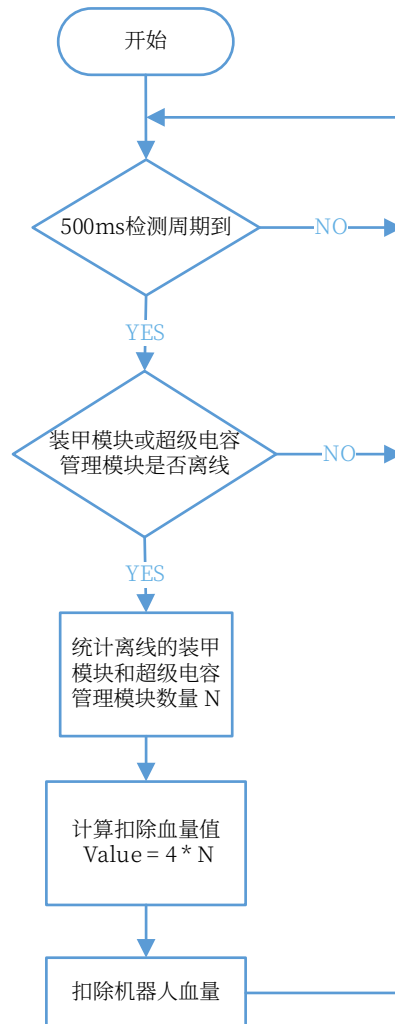
图 5-3 装甲模块和超级电容管理模块离线的扣血机制
