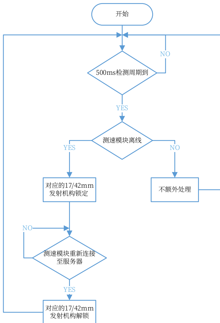
图 5-4 测速模块离线的断电机制
