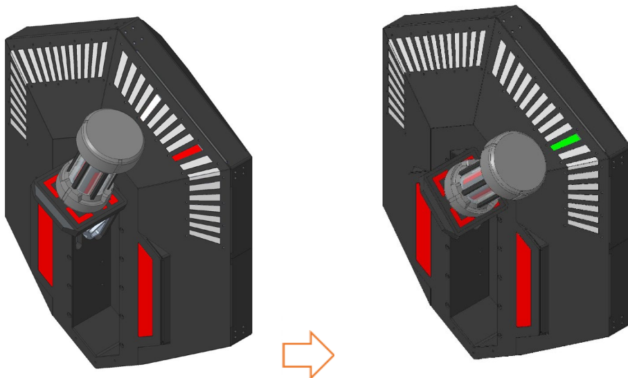
图 5-15 步骤 5 示意图
