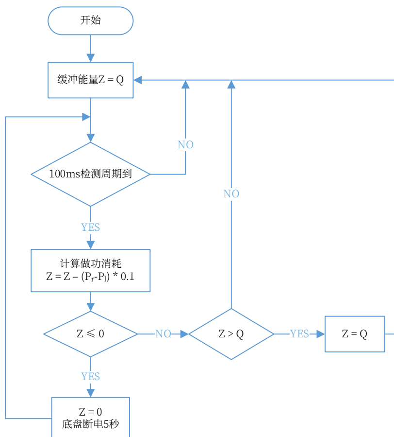
图 5-2 机器人底盘功率检测及超限惩罚机制
