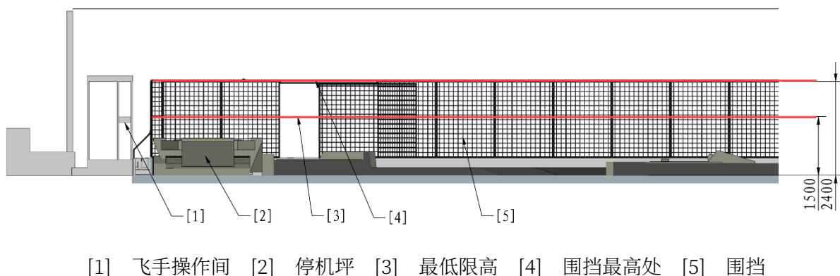
图 7-1 飞行高度限制示意图
