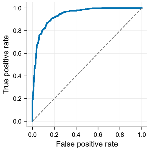
ROC, AUC = 0.939
