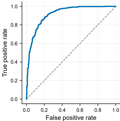
ROC, AUC = 0.916
