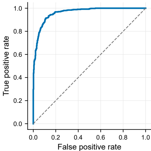
ROC, AUC = 0.961
