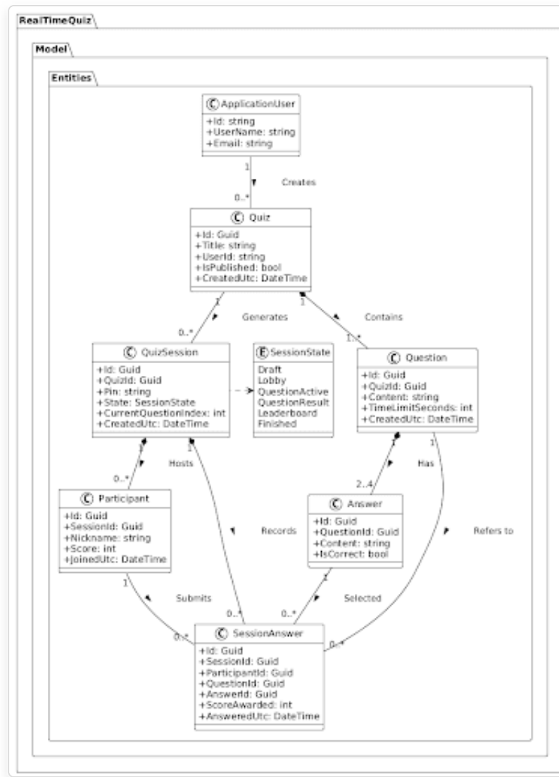
2. ábra - Osztály diagram
