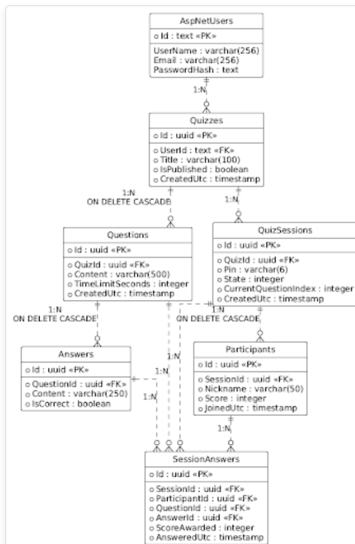
3. ábra - Adatbázis diagram
