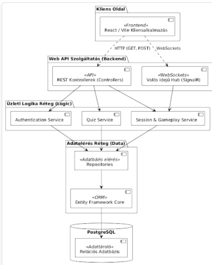
1. ábra - Komponens diagram
