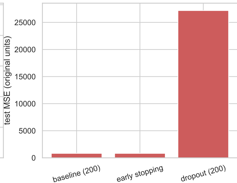
Test MSE
