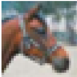
T:horse\nP:cat
