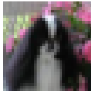
T:dog\nP:cat
