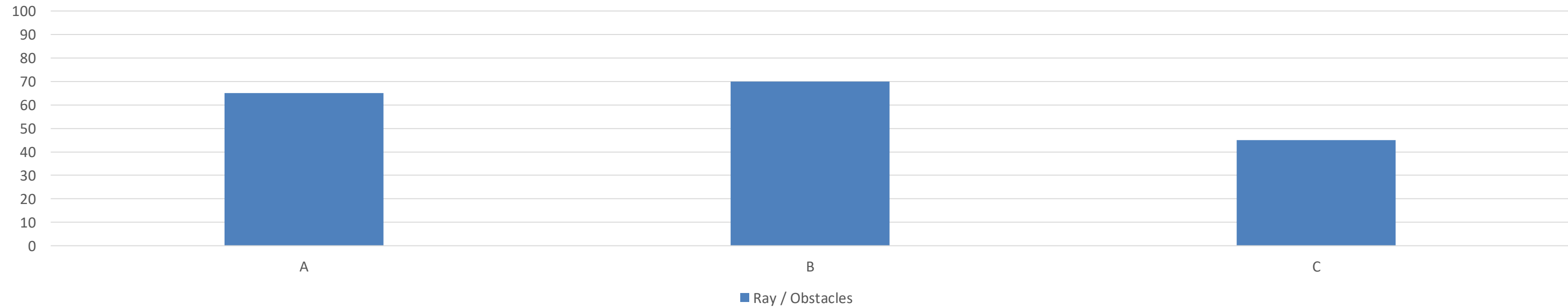
Visual Density
