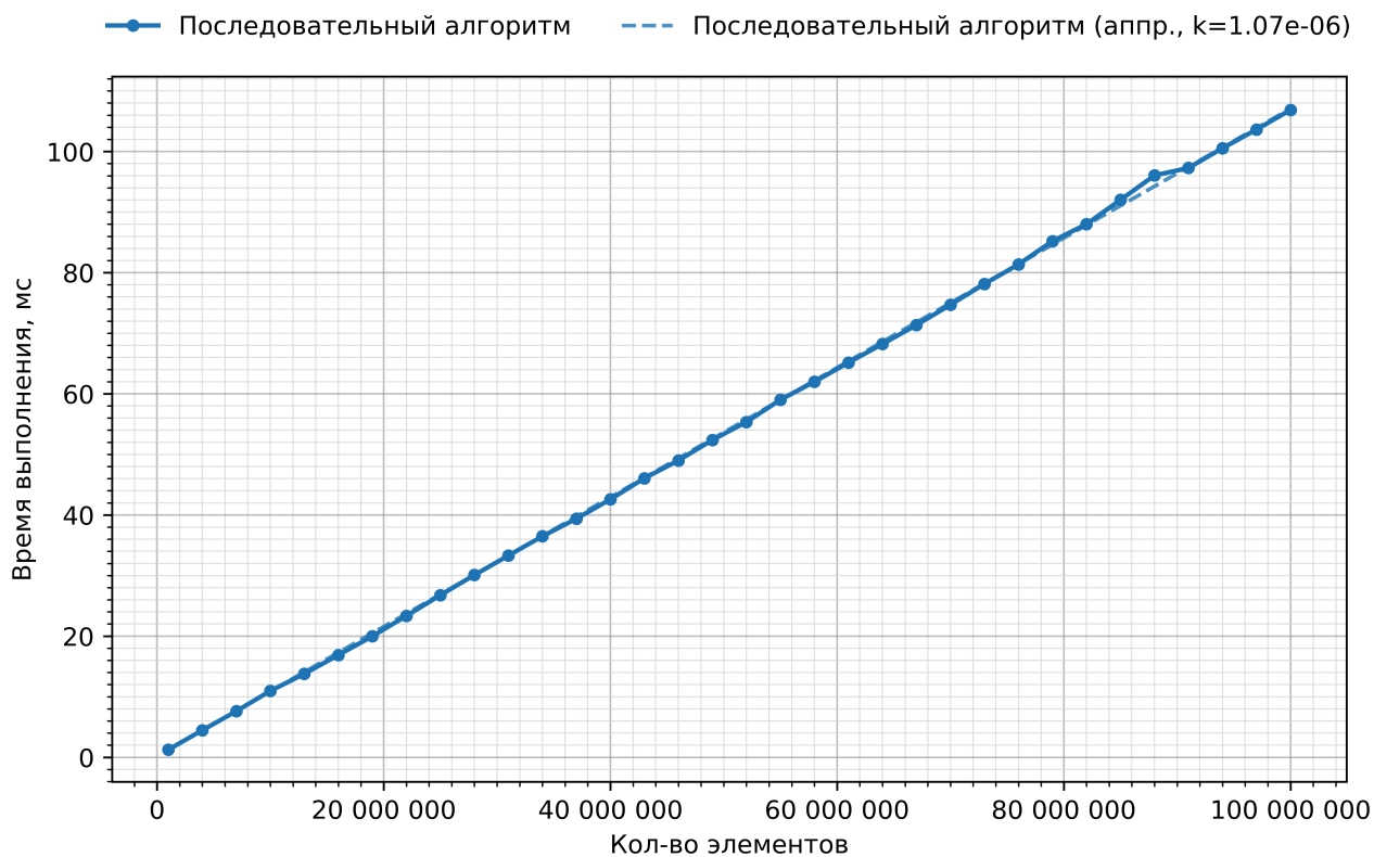
Рисунок 2 – График зависимости времени выполнения последовательного алгоритма от количества элементов в массиве
