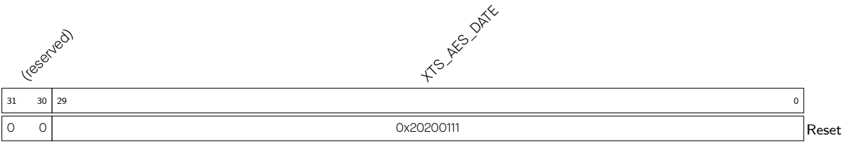
Register 23.9. XTS_AES_DATE_REG (0x005C)
