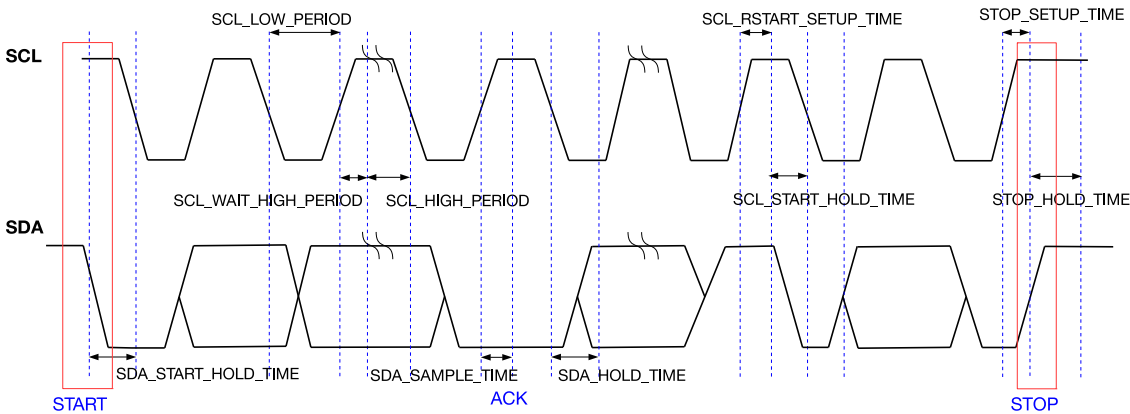
图 27.4-1. I2C 时序图
