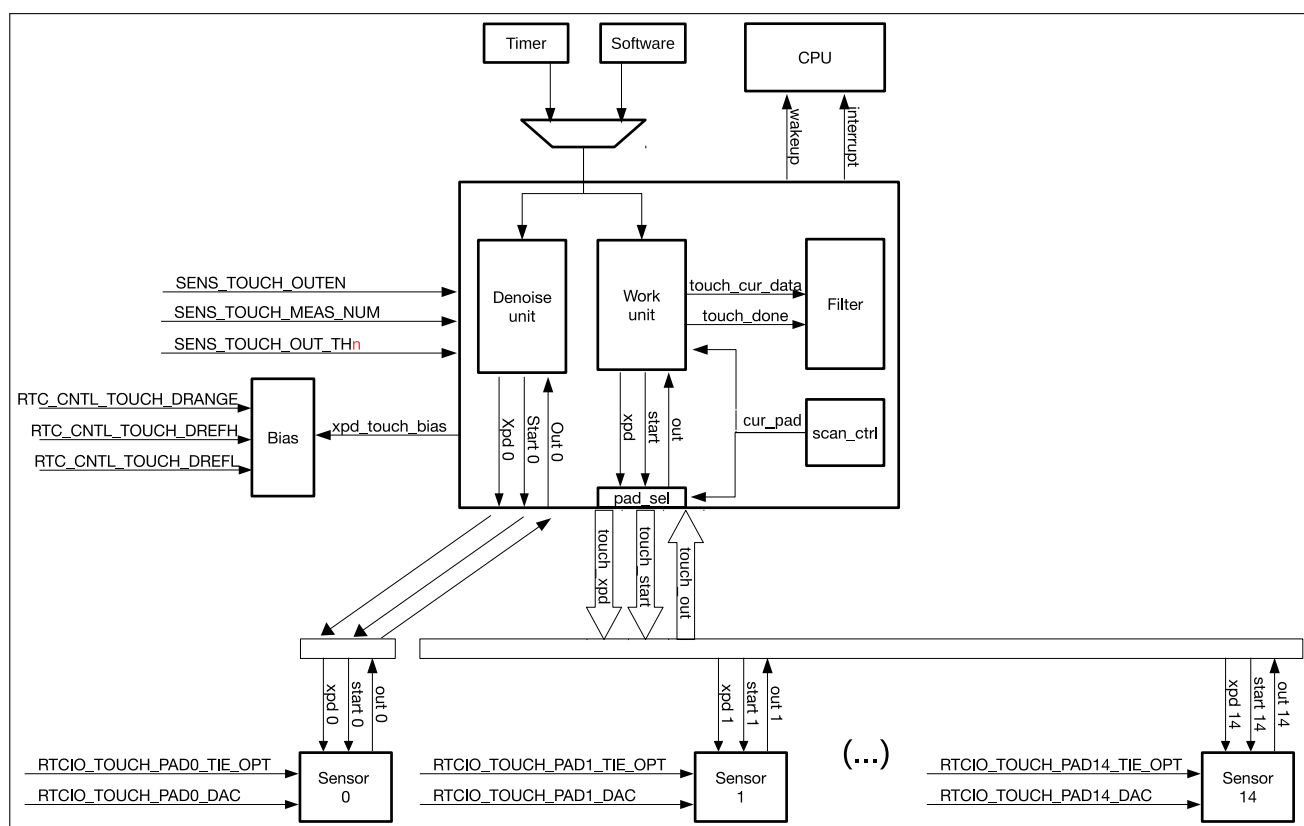
图 39.2-4. Touch FSM 的内部结构
