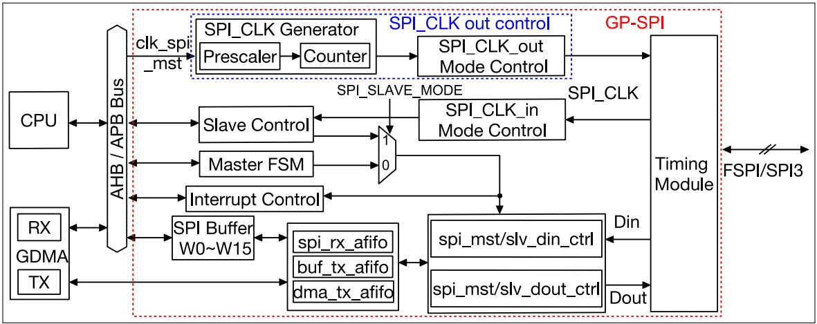
图 30.5-2. GP-SPI 功能块图
