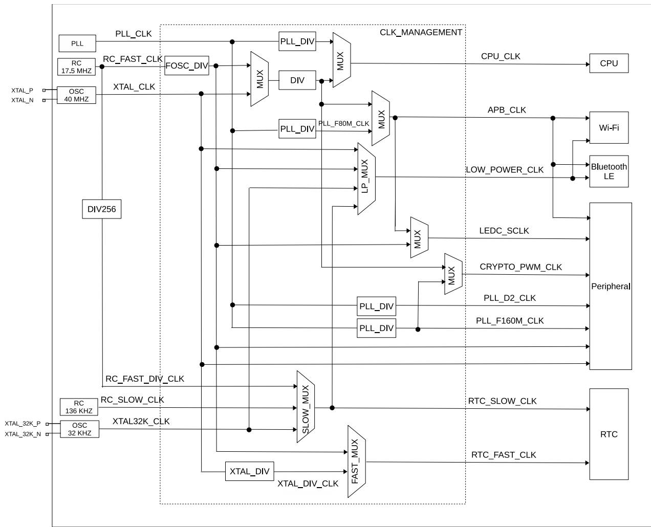
图 7.2-1. 系统时钟
