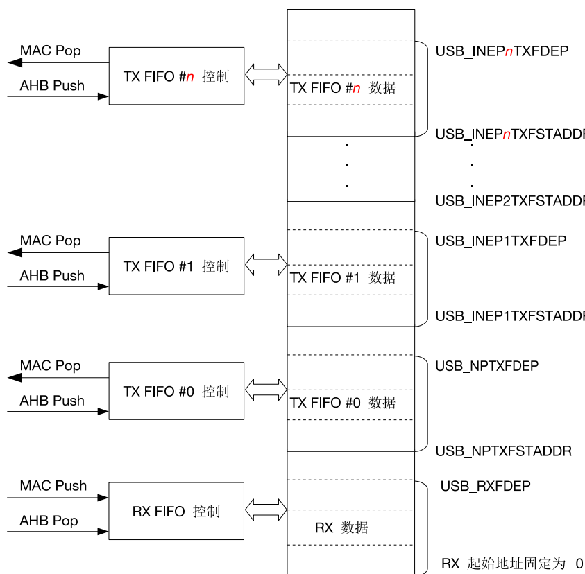
图 32.3-4. 设备模式 FIFO
