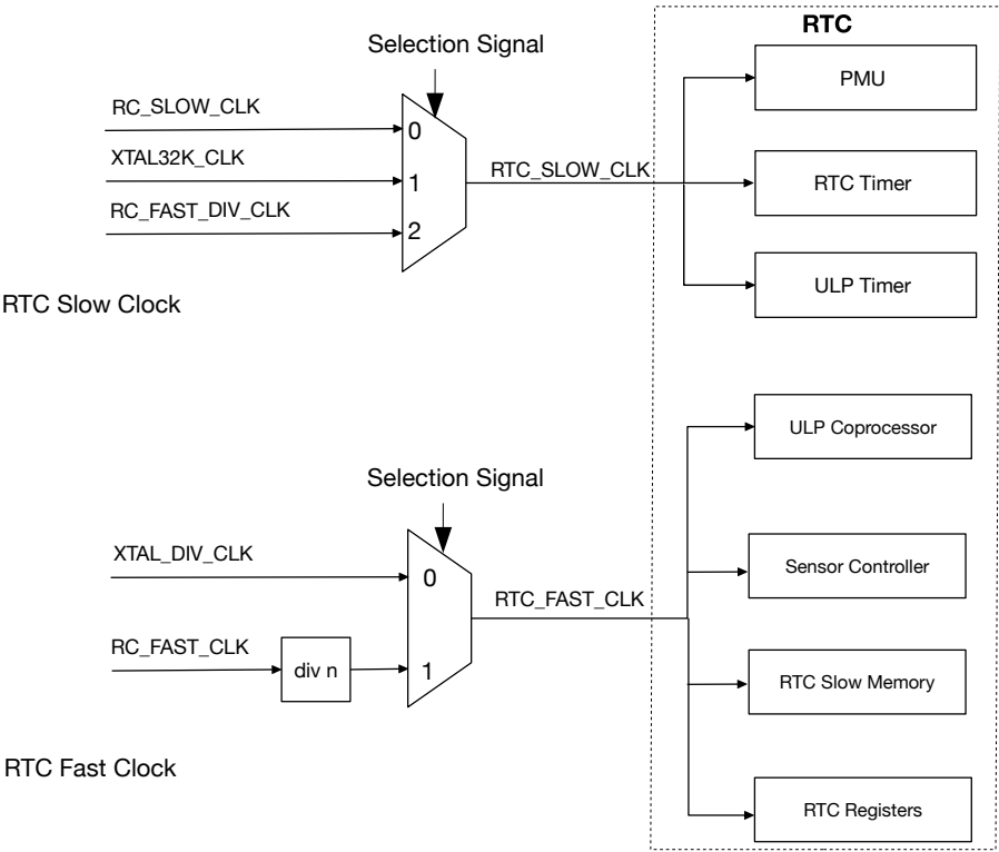
图 10.3-3. RTC 时钟
