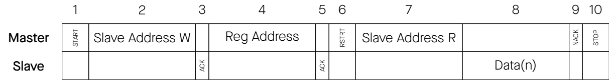
图 2.7-1. I2C 读操作
