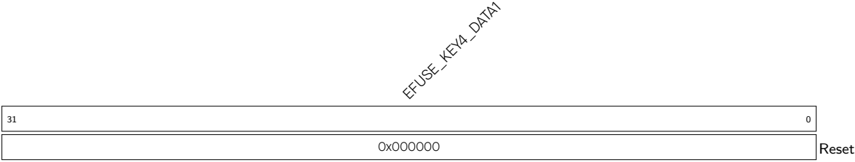
Register 5.73. EFUSE_RD_KEY4_DATA1_REG (0x0120)
