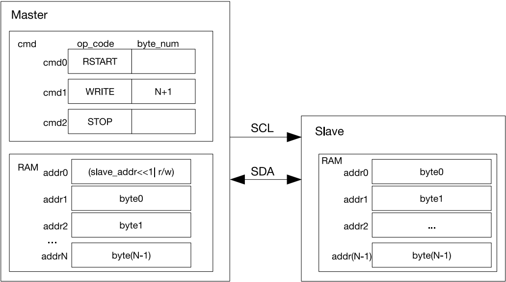
图 27.5-1. I2C 主机写 7 位寻址的从机
