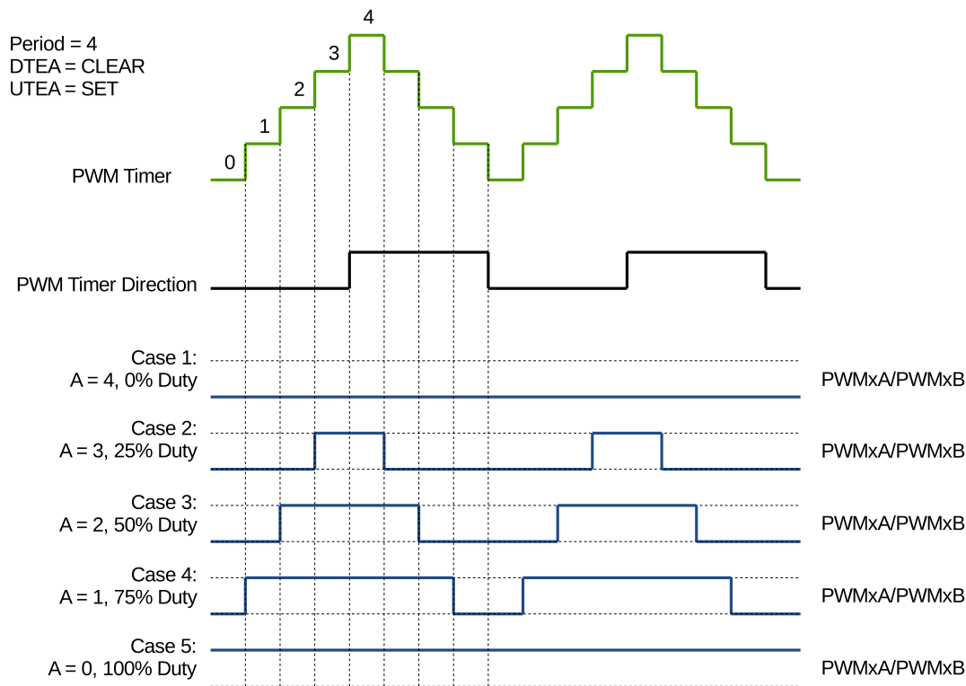
图 36.3-14. 递增递减模式下的对称波形
