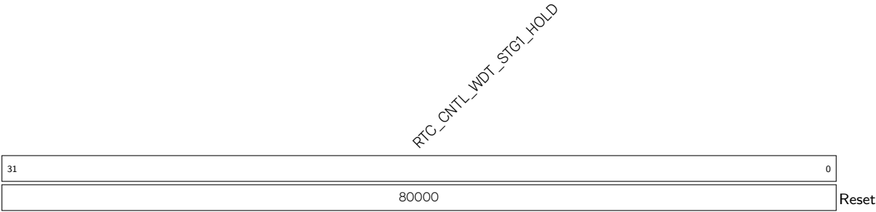
Register 10.34. RTC_CNTL_RTC_WDTCONFIG2_REG (0x00A0)
