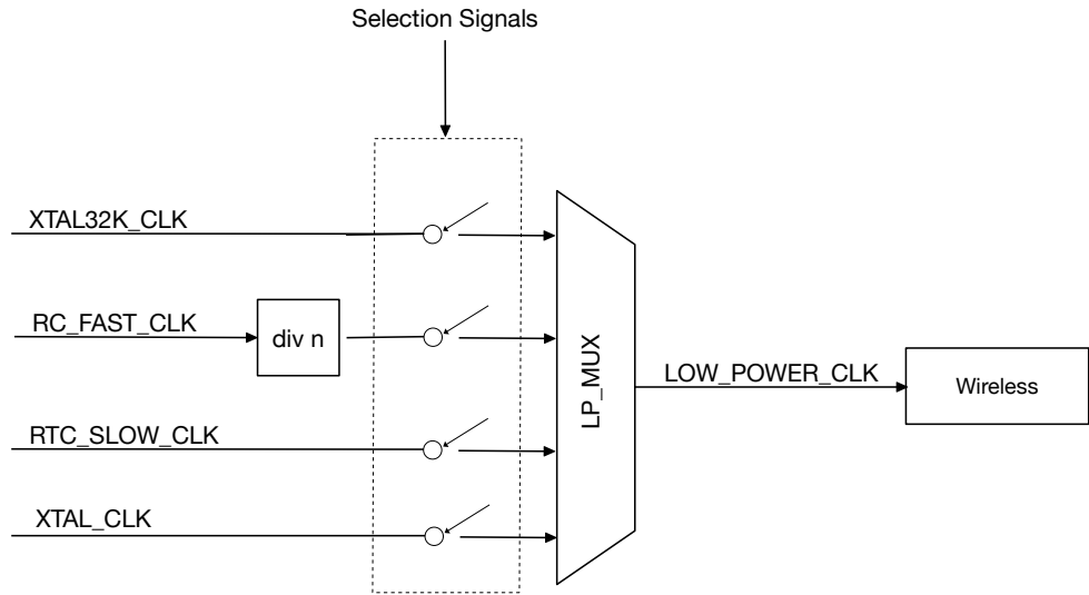
图 10.3-4. Wireless 时钟
