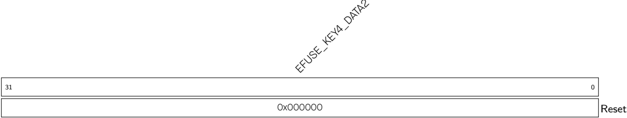
Register 5.74. EFUSE_RD_KEY4_DATA2_REG (0x0124)
