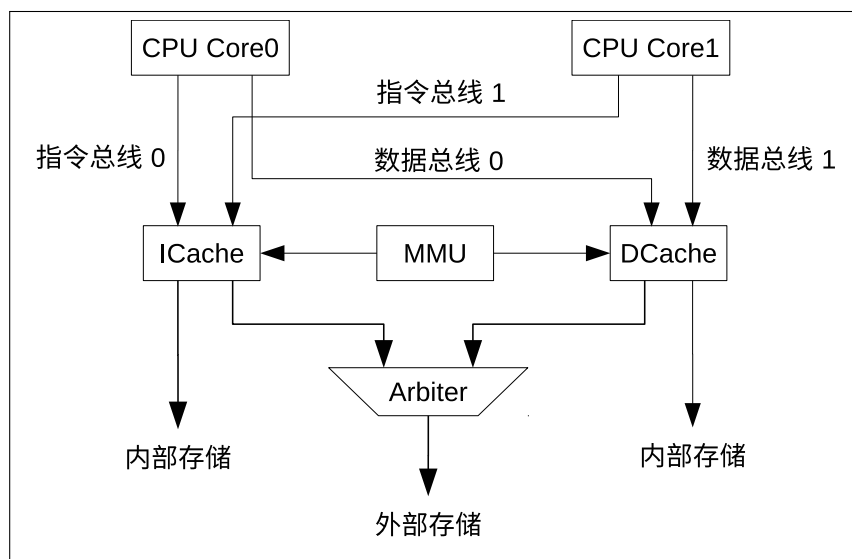
图 4.3-1. Cache 系统框图
