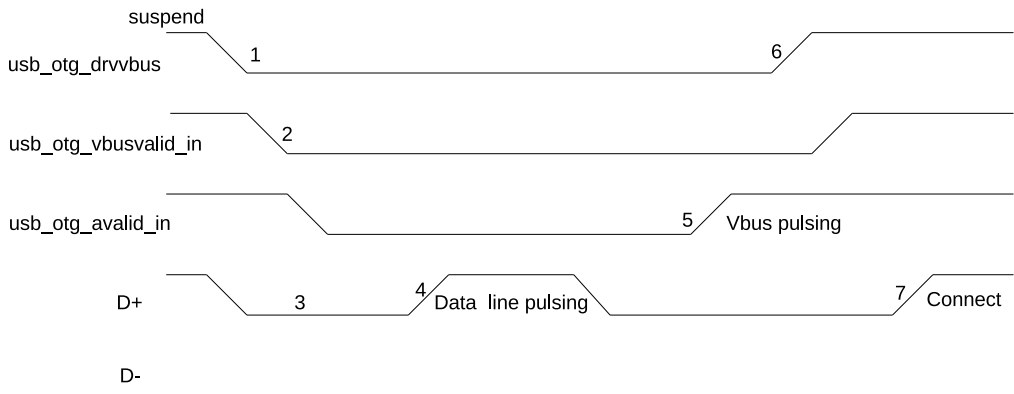
图 32.4-1. A 设备 SRP
