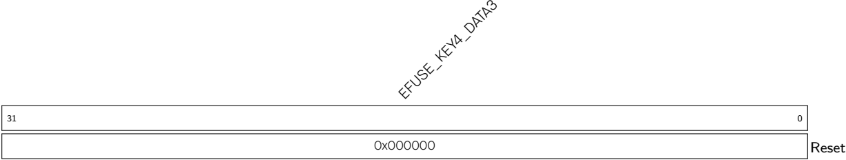
Register 5.75. EFUSE_RD_KEY4_DATA3_REG (0x0128)
