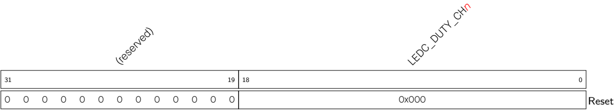
Register 35.5. LEDC_CH n _DUTY_REG ( n : 0-7) (0x0008+0x14* n )
