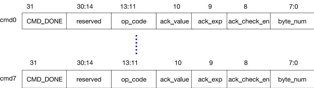
图 27.4-2. I2C 命令寄存器结构
