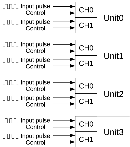
图 38.0-1. PCNT 框图
