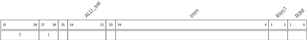
图 2.5-3. 指令类型 - 对指令立即值的 ALU 运算
