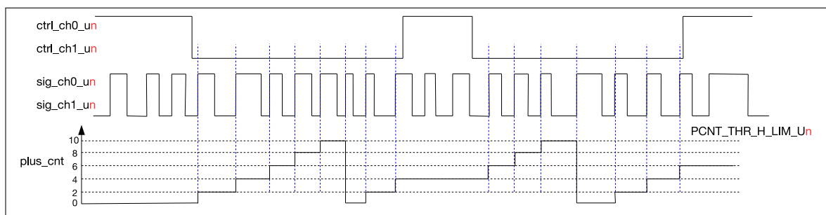
图 38.3-3. 双通道递增计数图
