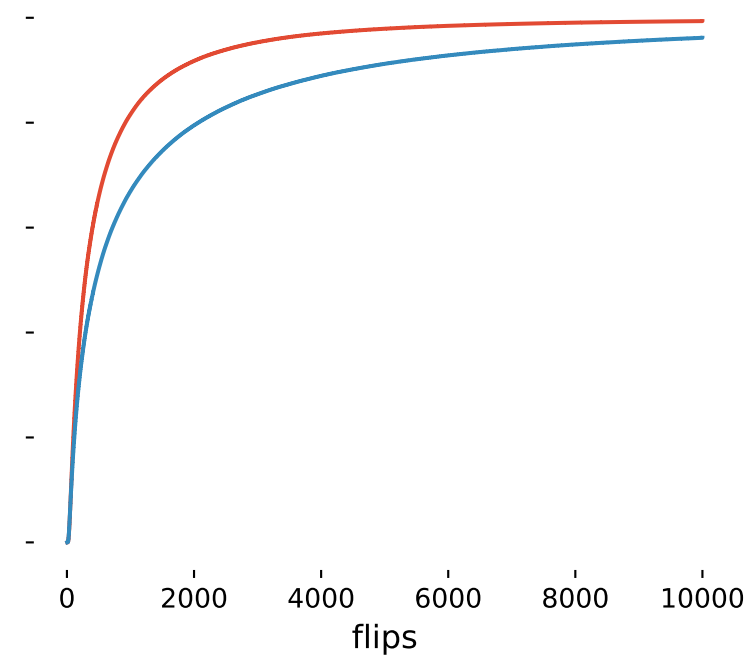
dataset = ruf50-218
