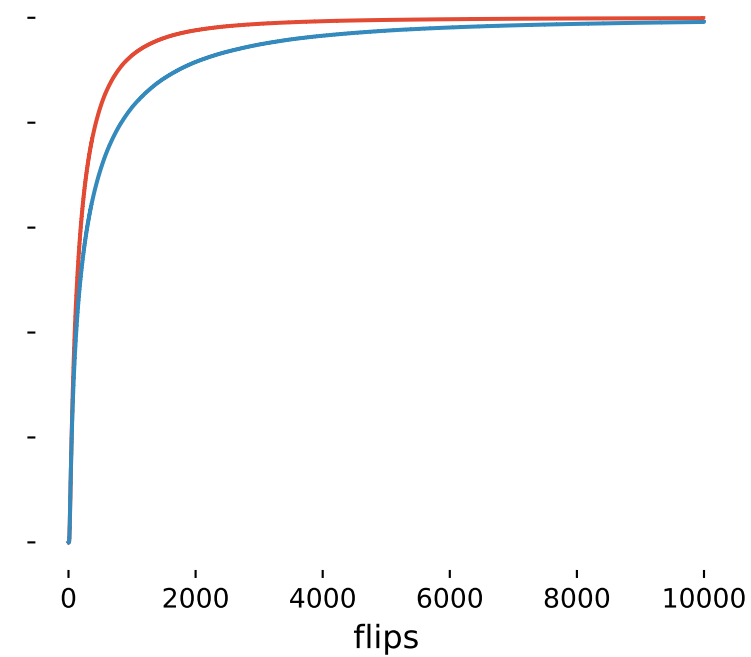
dataset = ruf36-157
