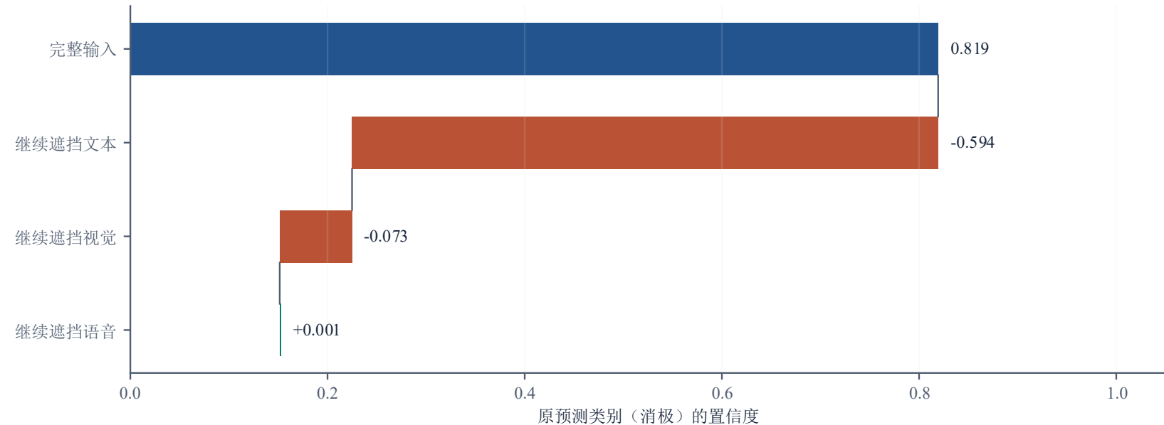
验证样本第6条：顺序模态消融
