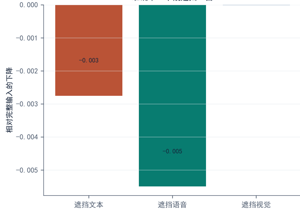
准确率：中段遮挡15窗
