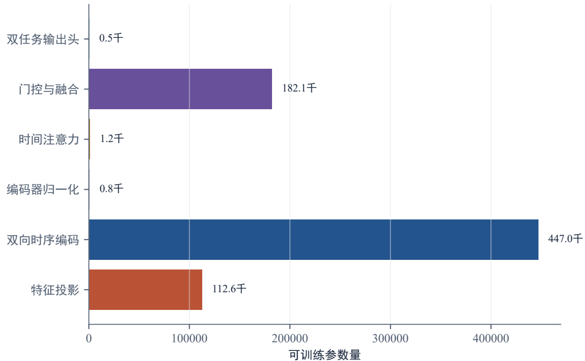
最终模型参数构成
