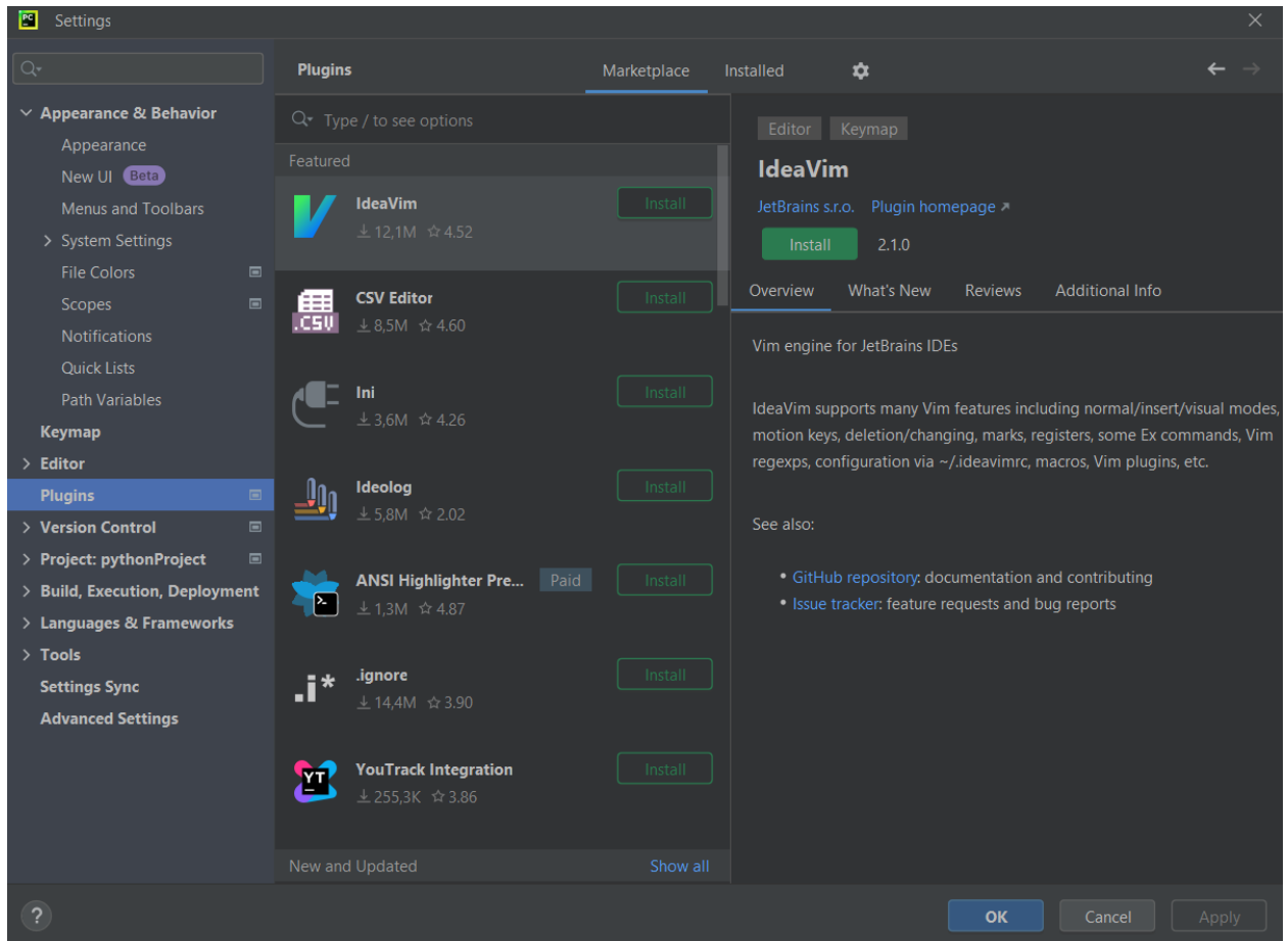
Рисунок 11 – Настройки -> плагины
