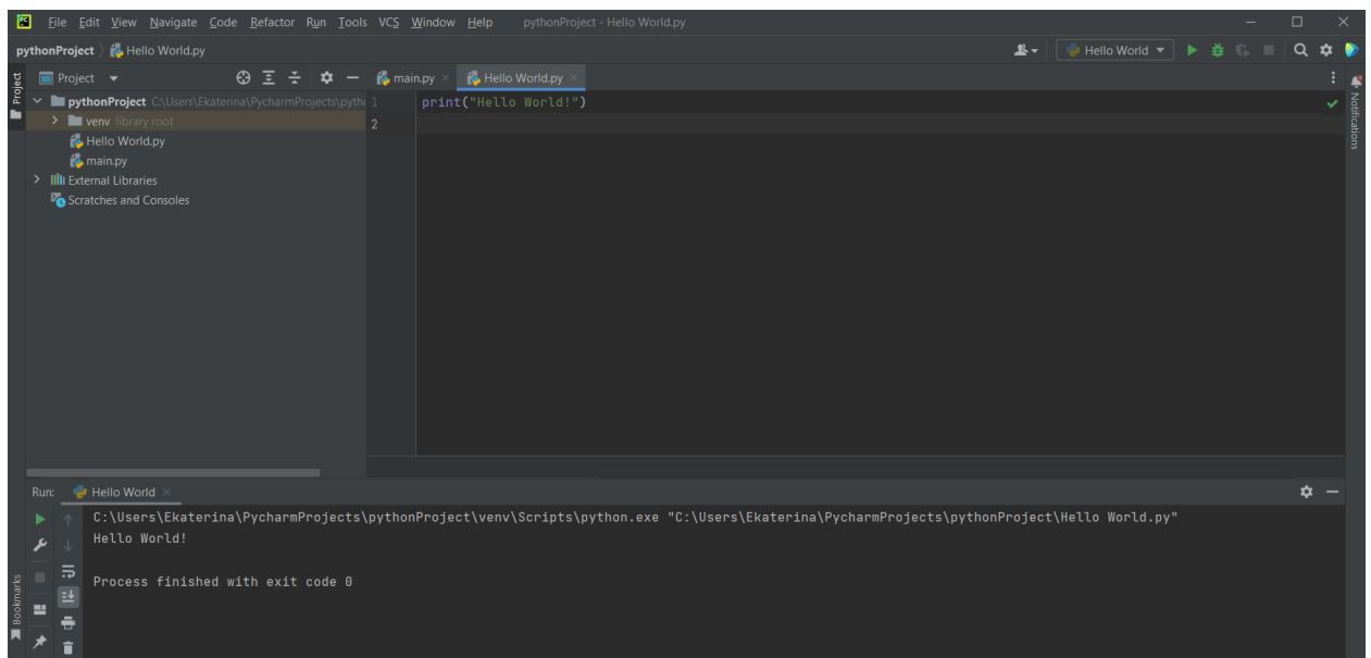
Рисунок 3 – выполнение программы
