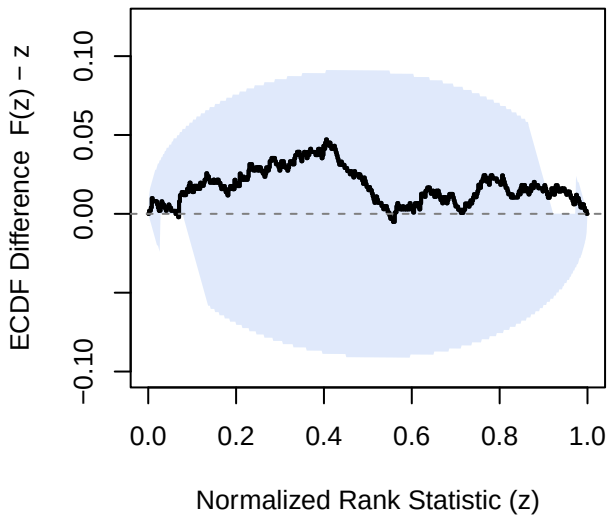
var - s.s
