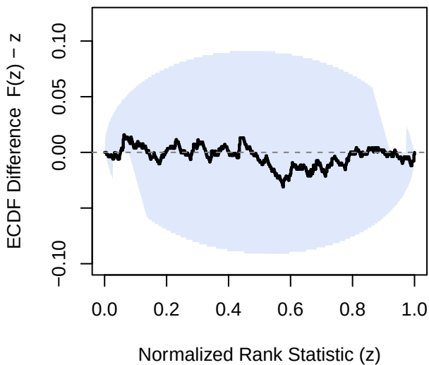
\mu - s
