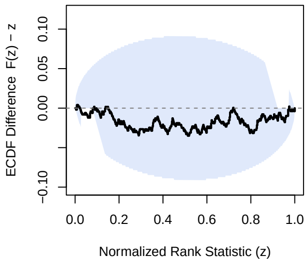
\mu - t_0
