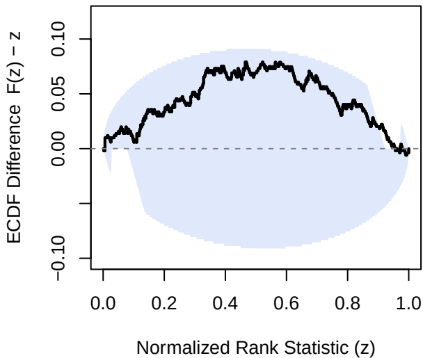
var - m.m
