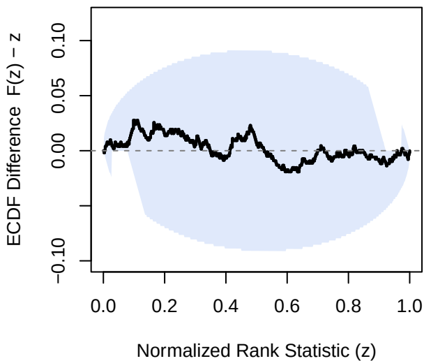
\mu - m
