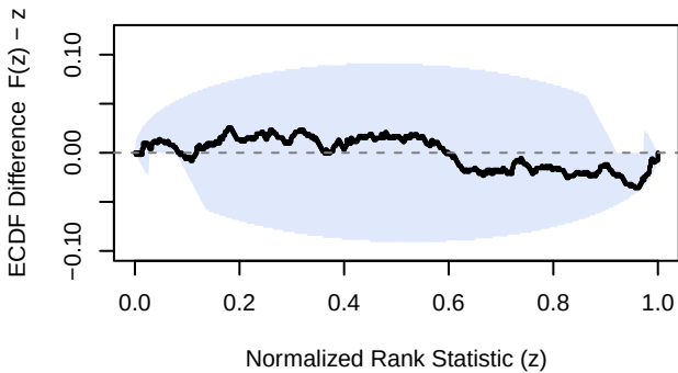
\mu - A
