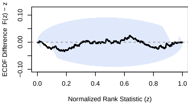
\mu - B
