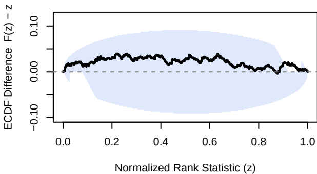
var - B.B
