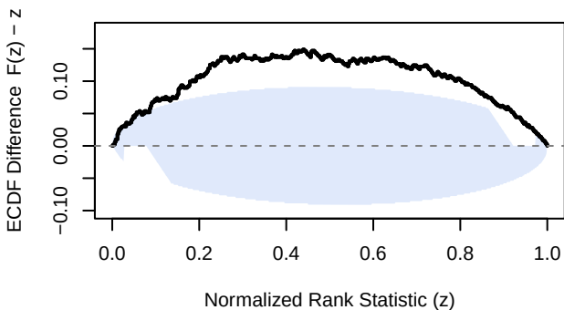
var - A.A
