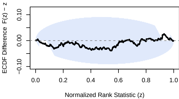
\mu - v
