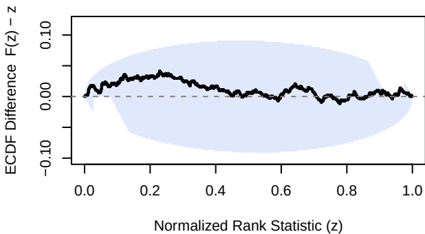
var - v.v
