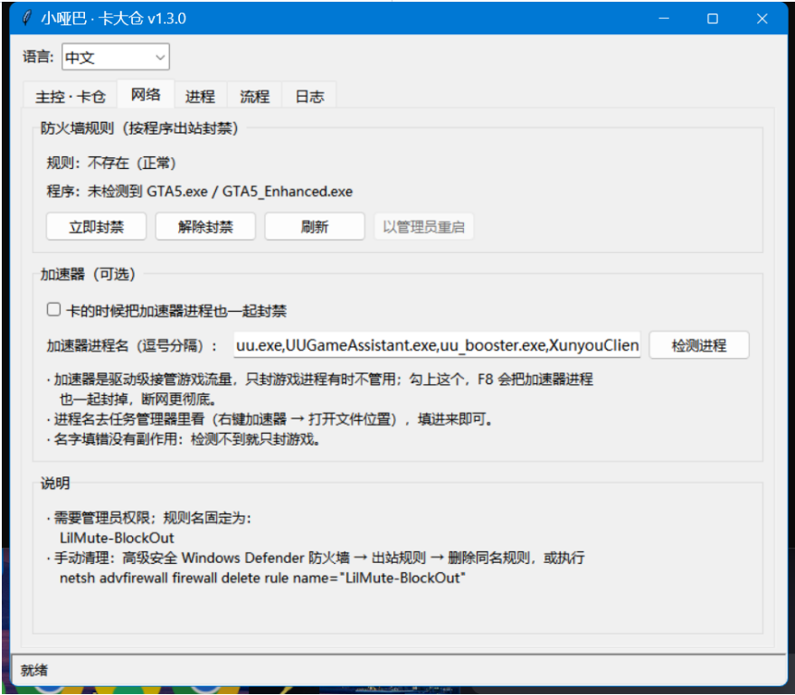
「网络」页：勾选后填进程名，点「检测进程」确认能找到
