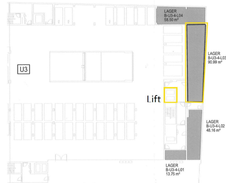
Grundriss des 3. Untergeschosses
