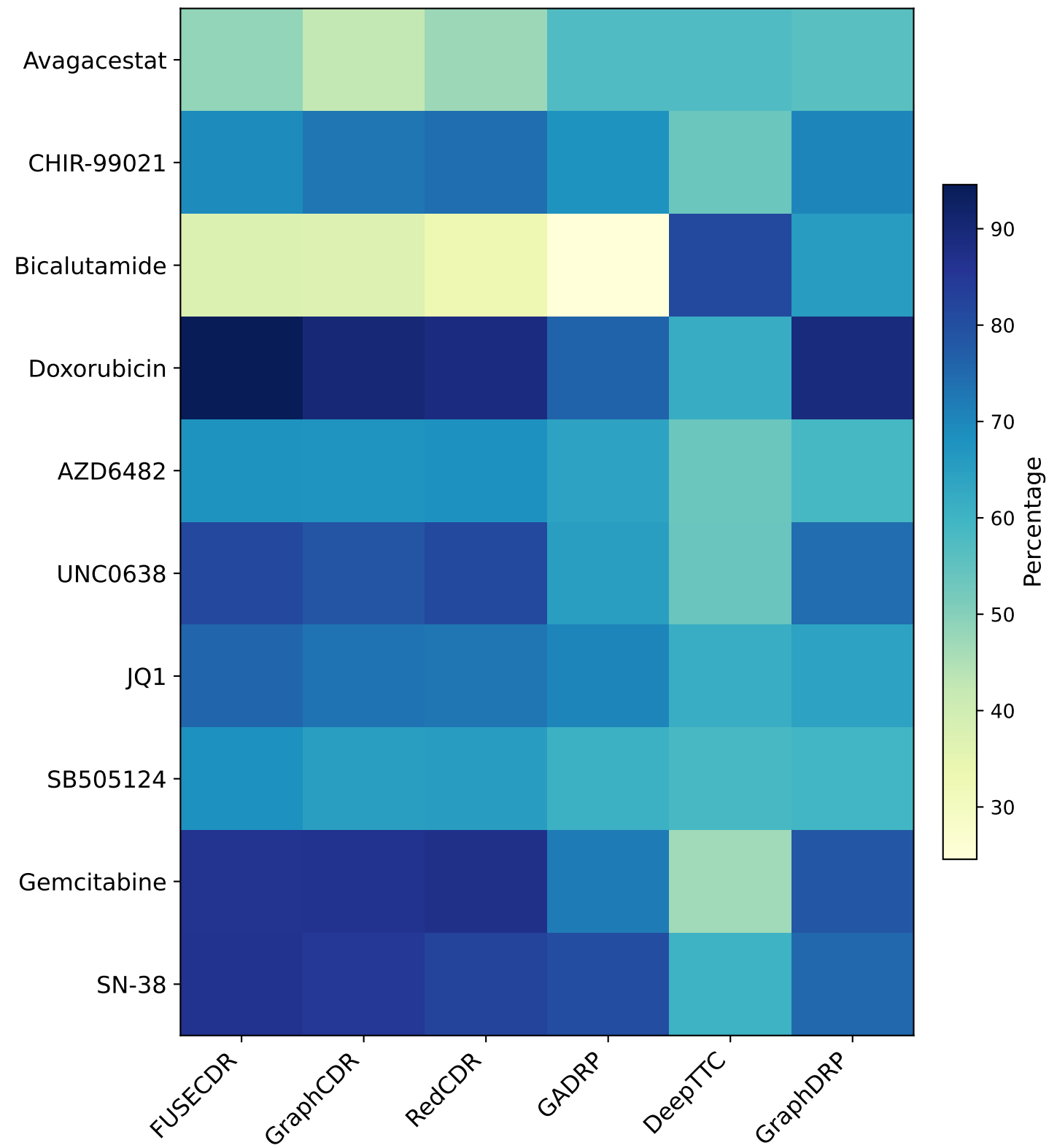
Drug-Level AUC
