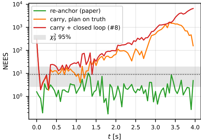
Estimator NEES
