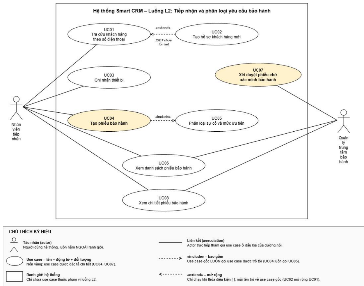
Hình 1. Use Case Diagram luồng L2 (file gốc: docs/usecase.drawio)
