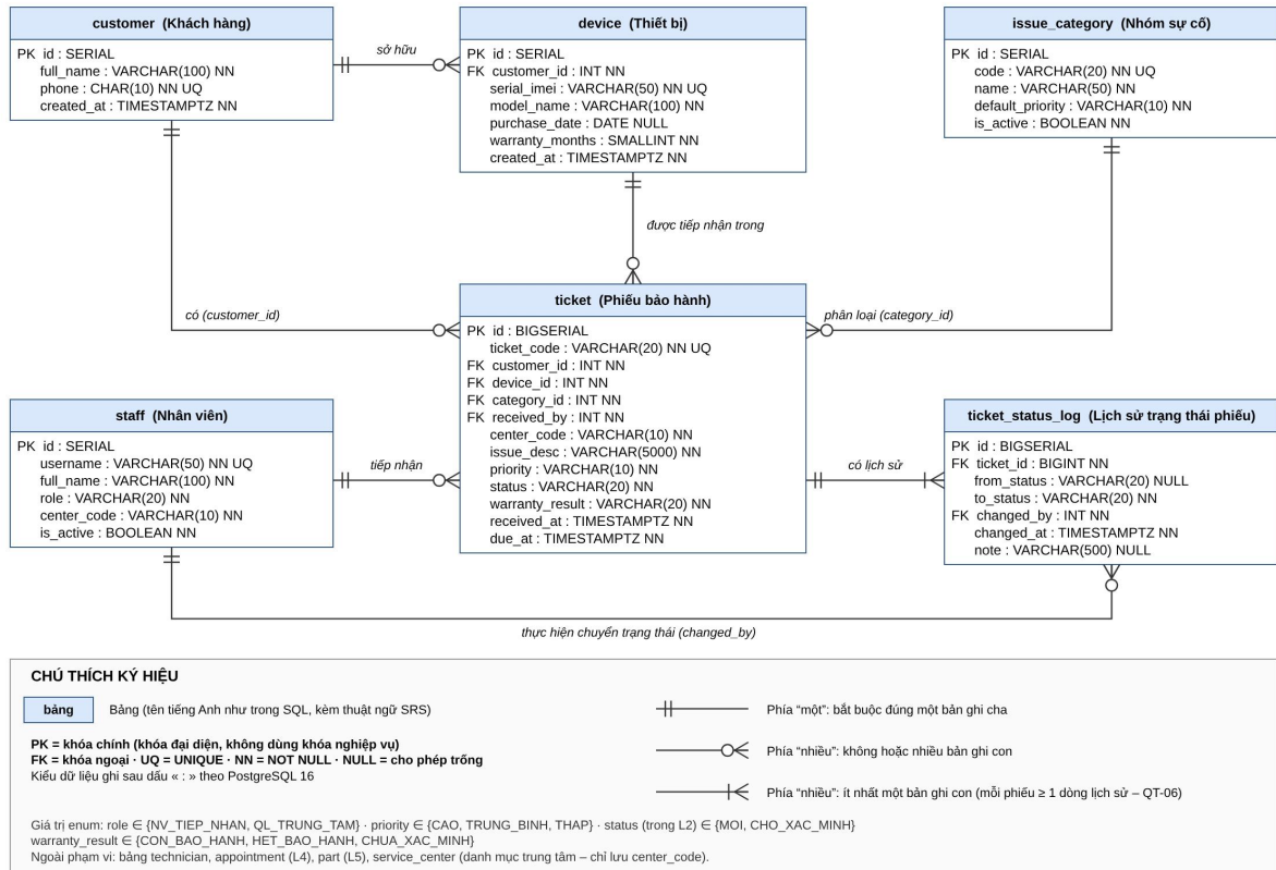
Hình 3. ERD luồng L2 – 6 bảng (file gốc: docs/erd.drawio)
