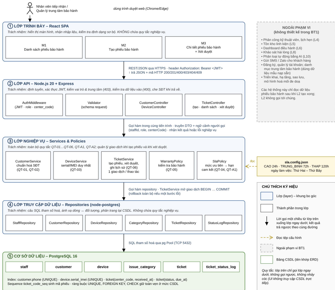
Hình 2. Kiến trúc phân lớp cho luồng L2 (file gốc: docs/architecture.drawio)
