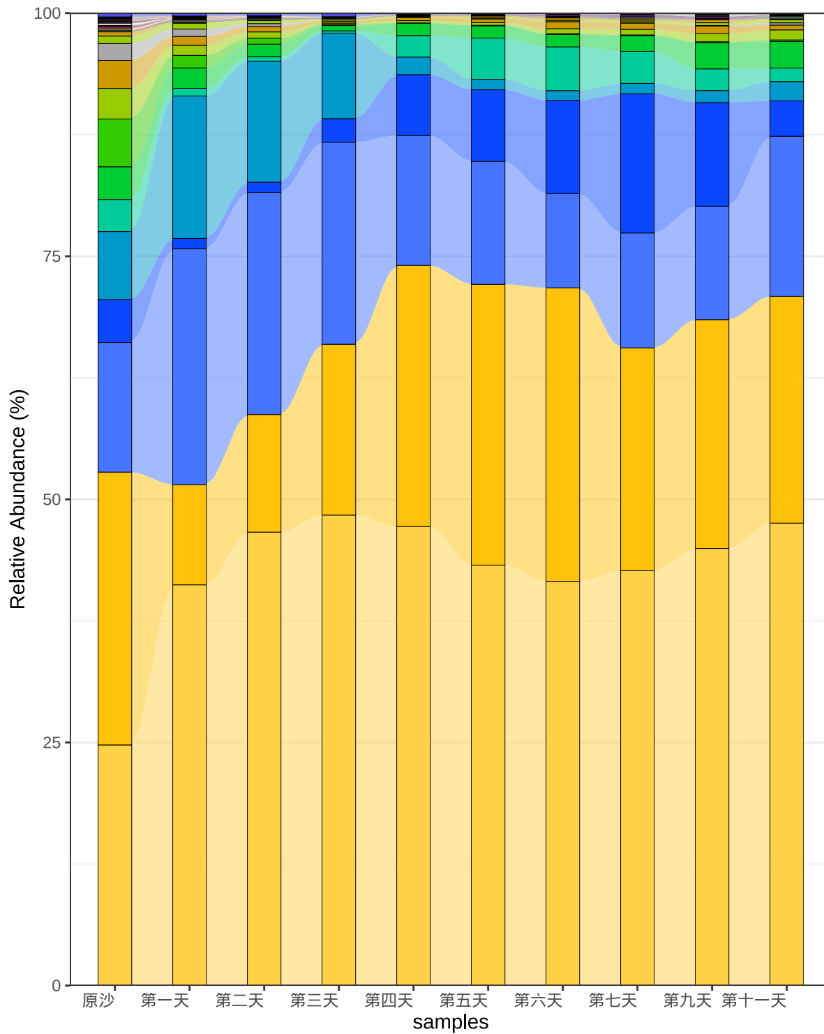
细菌组成变化情况
