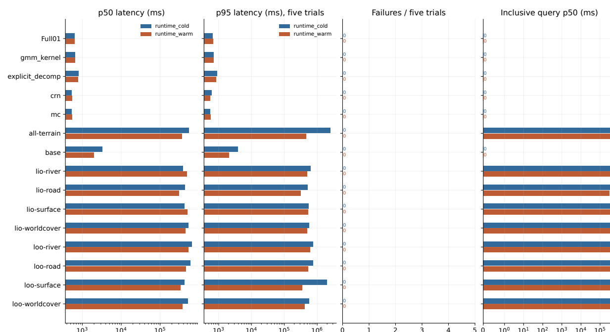
图 7: 原 15 对象 provider 冷 / 热延迟 p50/p95 (毫秒) 与失败数。第四面板从原试验记录取包含在总耗时中的地形 I/O / 查询中位毫秒; 无地形阶段为零, 不是额外成本。各条件五次, 15 次预热排除于分位数, 而不是排除记录中断暴露试验。provider 冷不是 OS 缓存冷; 查询包含于 rollout, 五次不估计稳定部署尾延迟。
