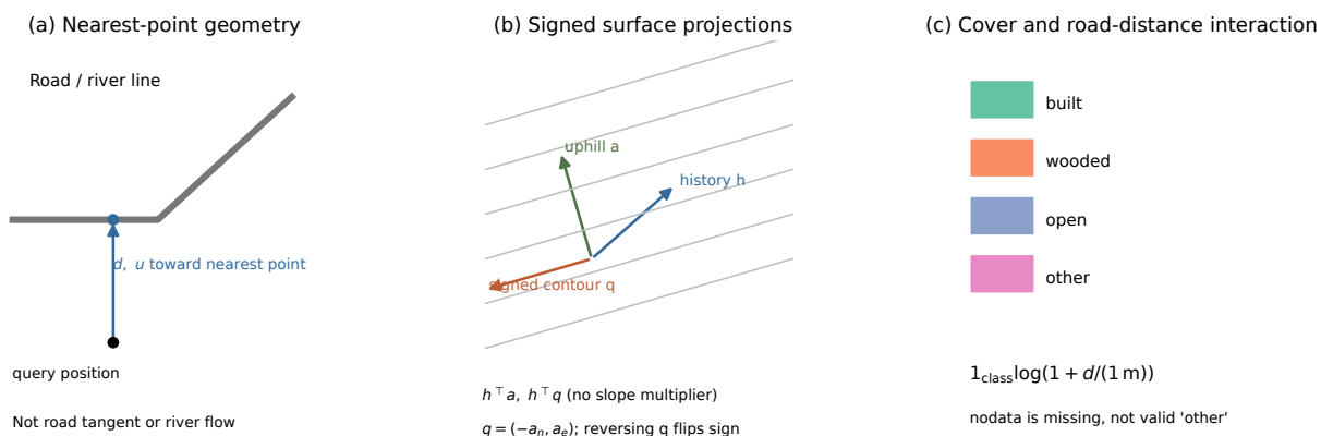
图 1: 几何示意而非真实路线。左：道路 / 河流最近点、距离及指向该点的方向，不是切线或流向。中：带符号历史 h 、上坡 a 、等高线 q 的不同点积与坡度大小。右：覆盖类别和保留道路距离的组合；无效查询不是有效“其他”覆盖类。正文列明排除的道路类别。图内英文标签与本题注逐项对应。
