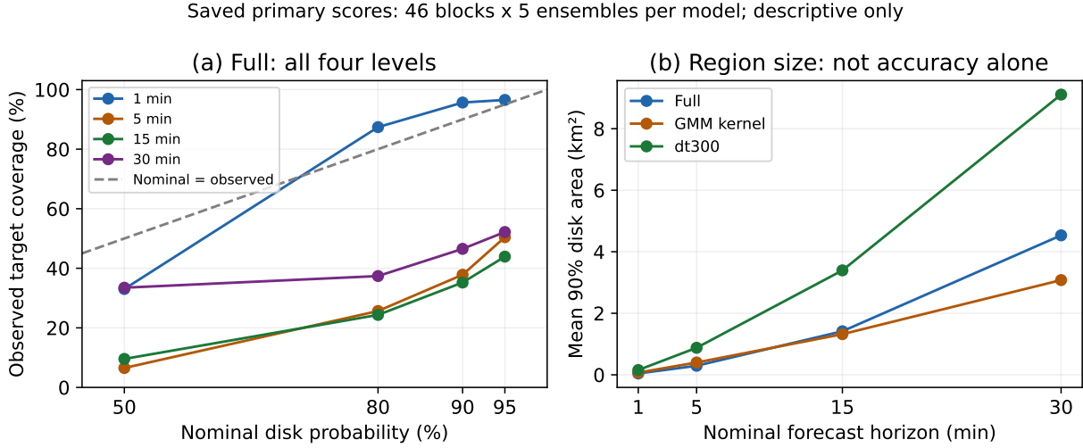
图 15: 已保存的校准与区域大小诊断, 不是新增实验。左: Full 各时域的实际覆盖对名义概率, 对角虚线表示名义一致。右: 此前三个模型的 90% 预测圆平均面积。连线仅在四个已测水平或时域间引导视线, 没有评价中间目标、整路径联合覆盖或新增统计检验。
