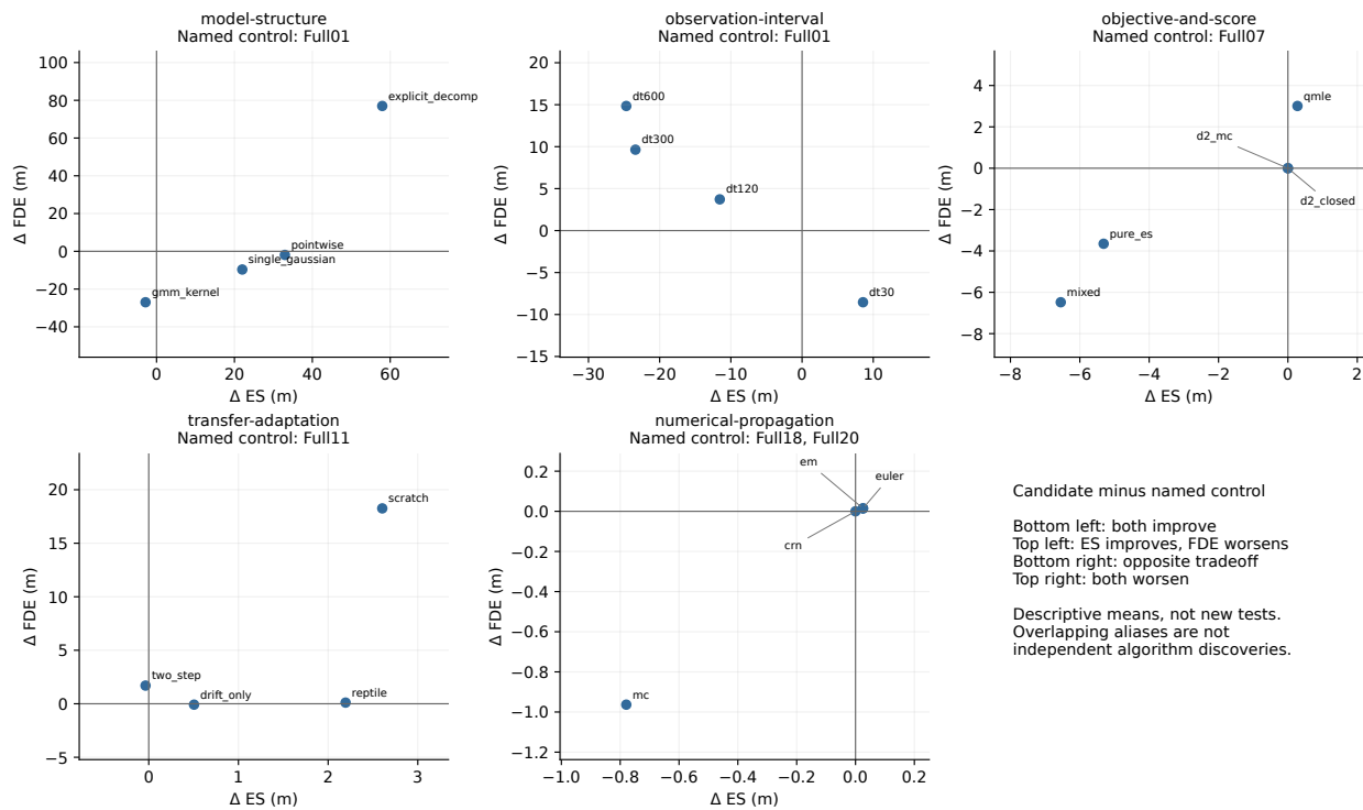
图 3: 全部 21 项候选减具名对照: 加权 ES 与均值位置 FDE (米), 两轴均负差有利。分面保留原家族, 各 Full 对照不合并。这是配对均值描述, 不是新联合检验或 Pareto 排名。
