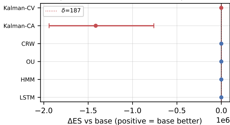
(d) paired verdict (block bootstrap B=2000)
