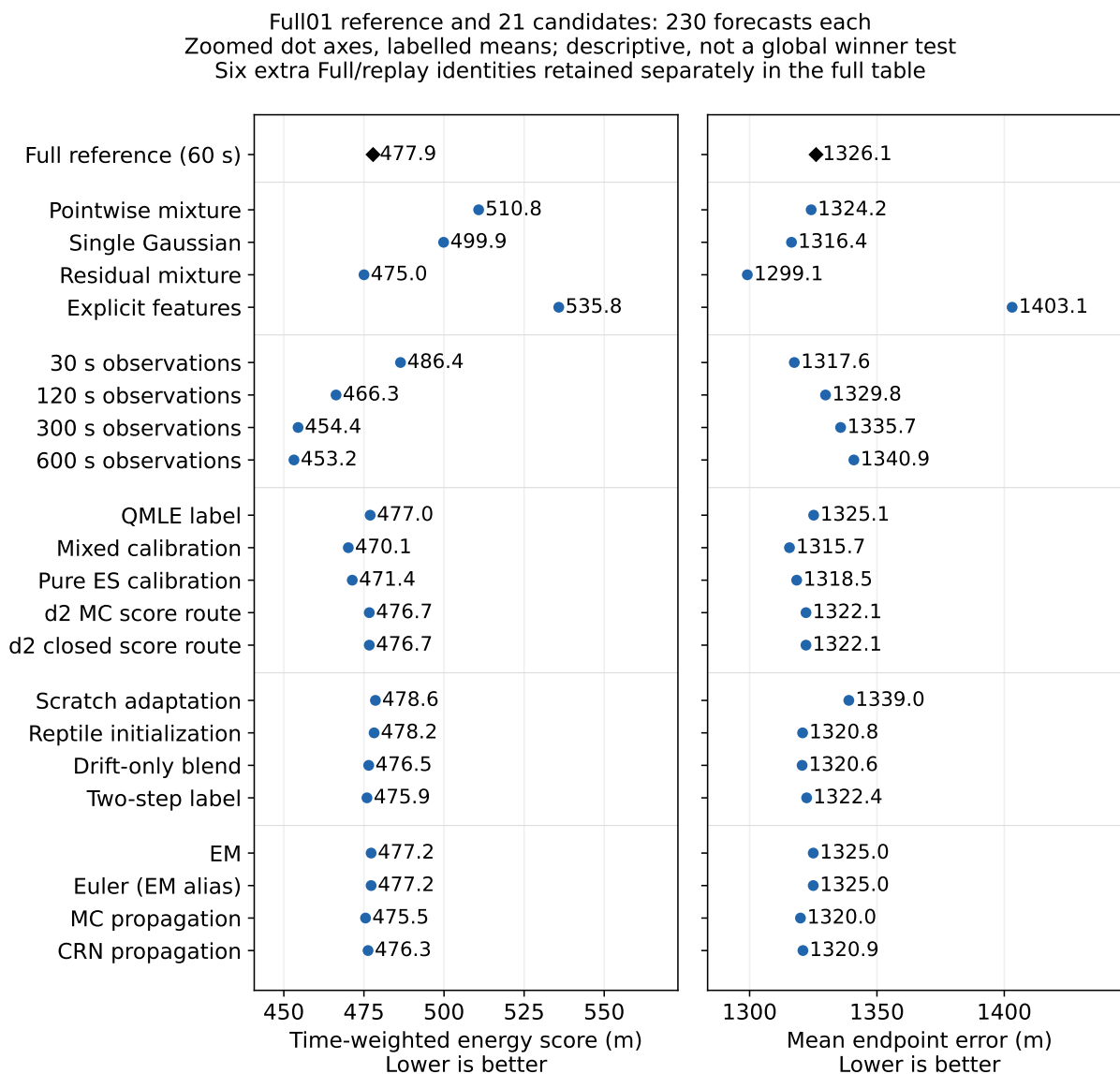
图 3: Full01 参考与全部 21 个候选, 以数值标注保存的绝对 ES 与终点误差均值, 单位米。两侧点图横轴均已放大, 越低越好; 点间距离不是配对效应估计。观测变体按间隔递增排列。六个额外 Full / replay 角色仅在本图省略, 仍分别保留于表 53, 不平均。每行完整使用 230 项预测; 评分路线和别名不是独立算法。这是描述图, 不是全局最佳者检验。
