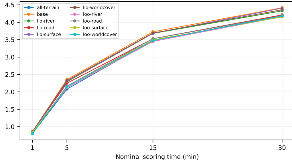
95% region area (m^2)
