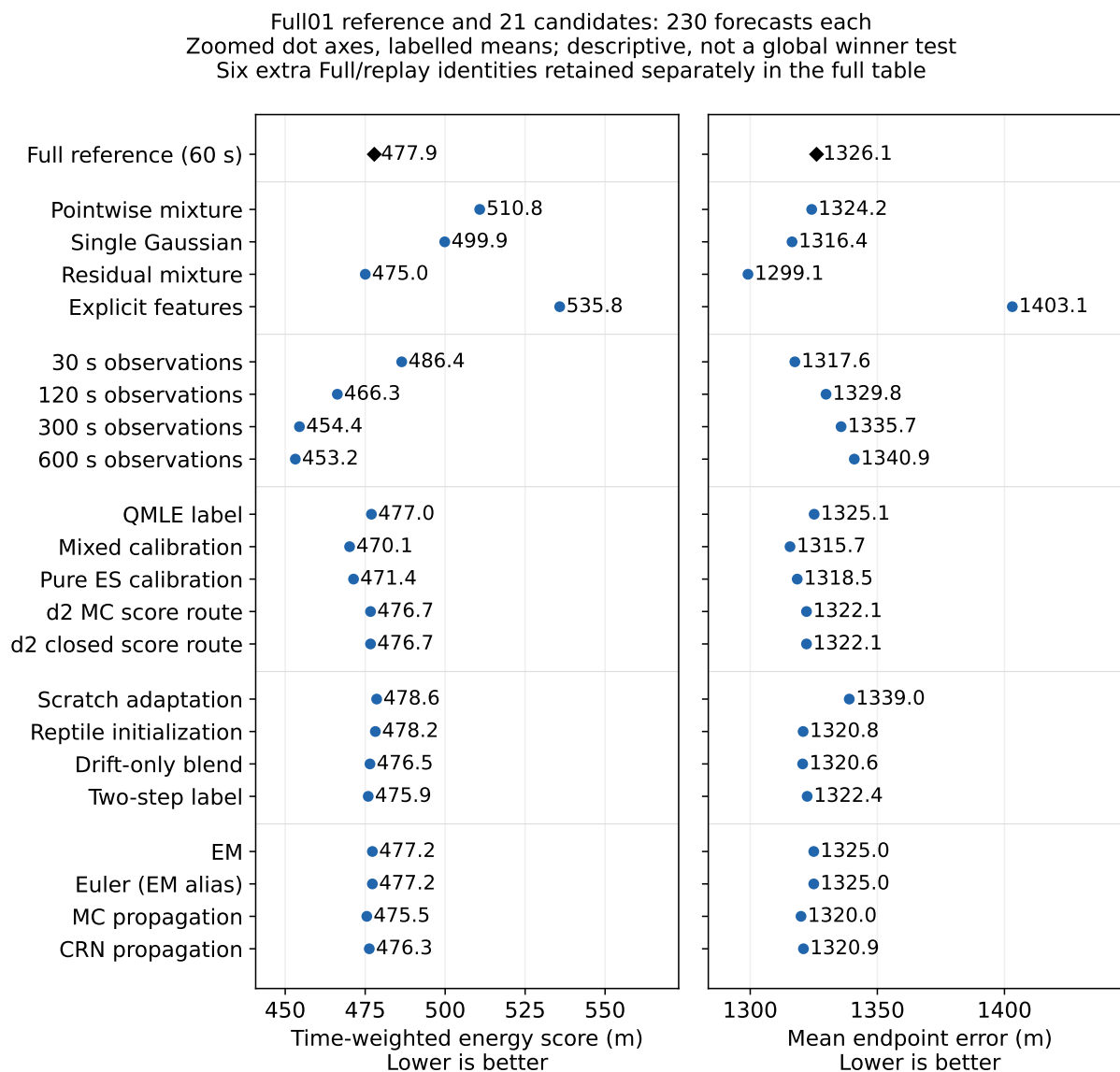
图 3: Full01 参考与全部 21 个候选, 以数值标注保存的绝对 ES 与终点误差均值, 单位米。两侧点图横轴均已放大, 越低越好; 点间距离不是配对效应估计。观测变体按间隔递增排列。六个额外 Full / replay 角色仅在本图省略, 仍分别保留于表 51, 不平均。每行完整使用 230 项预测; 评分路线和别名不是独立算法。这是描述图, 不是全局最佳者检验。
