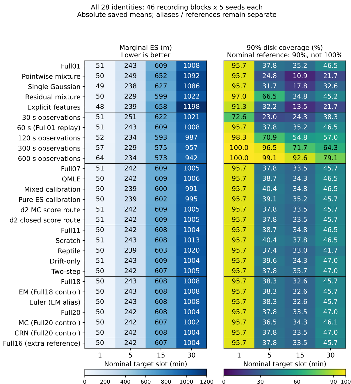
图 4: 全部 28 个主组保存配置在四个名义目标时域的概览; 没有新增中间时刻预测。左: 边际 ES (米), 越低越好。右: 名义 90% 预测圆的实际覆盖率 (%); 校准参考是 90% 而不是 100%, 本图不显示区域大小。每格平均同一 46 块、五个种子。概览 ES 舍入到整数米, 覆盖率保留一位小数; 完整精度和全部角色保留于保存投影及表 52。行按登记家族而非性能排序; 别名与不同 Full 对照不合并, 舍入相似不证明等价。这是描述展示, 不是新增逐时域检验或最终资格。
