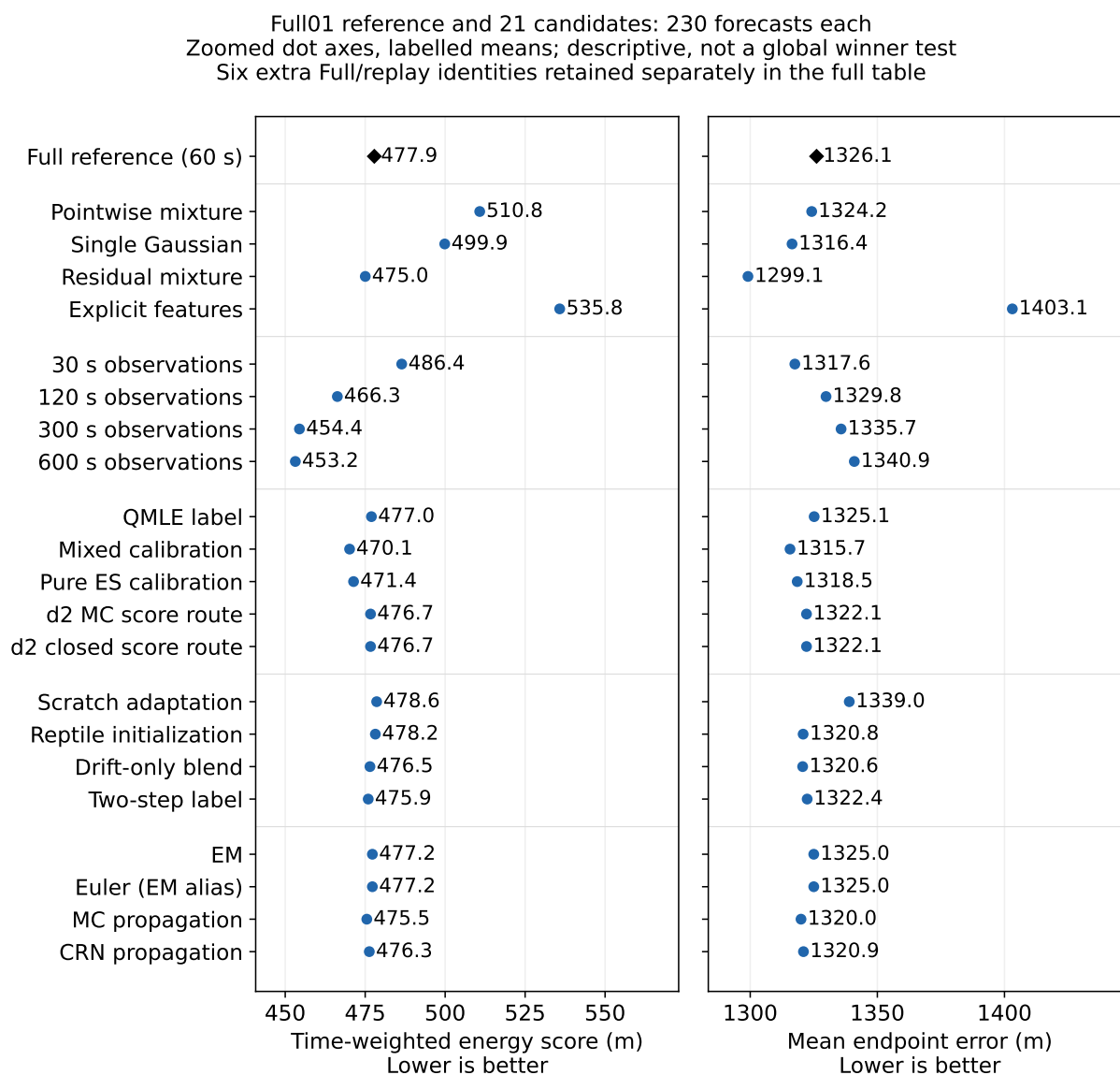
图 3: Full01 参考与全部 21 个候选, 以数值标注保存的绝对 ES 与终点误差均值, 单位米。两侧点图横轴均已放大, 越低越好; 点间距离不是配对效应估计。观测变体按间隔递增排列。六个额外 Full / replay 角色仅在本图省略, 仍分别保留于表 48, 不平均。每行完整使用 230 项预测; 评分路线和别名不是独立算法。这是描述图, 不是全局最佳者检验。
