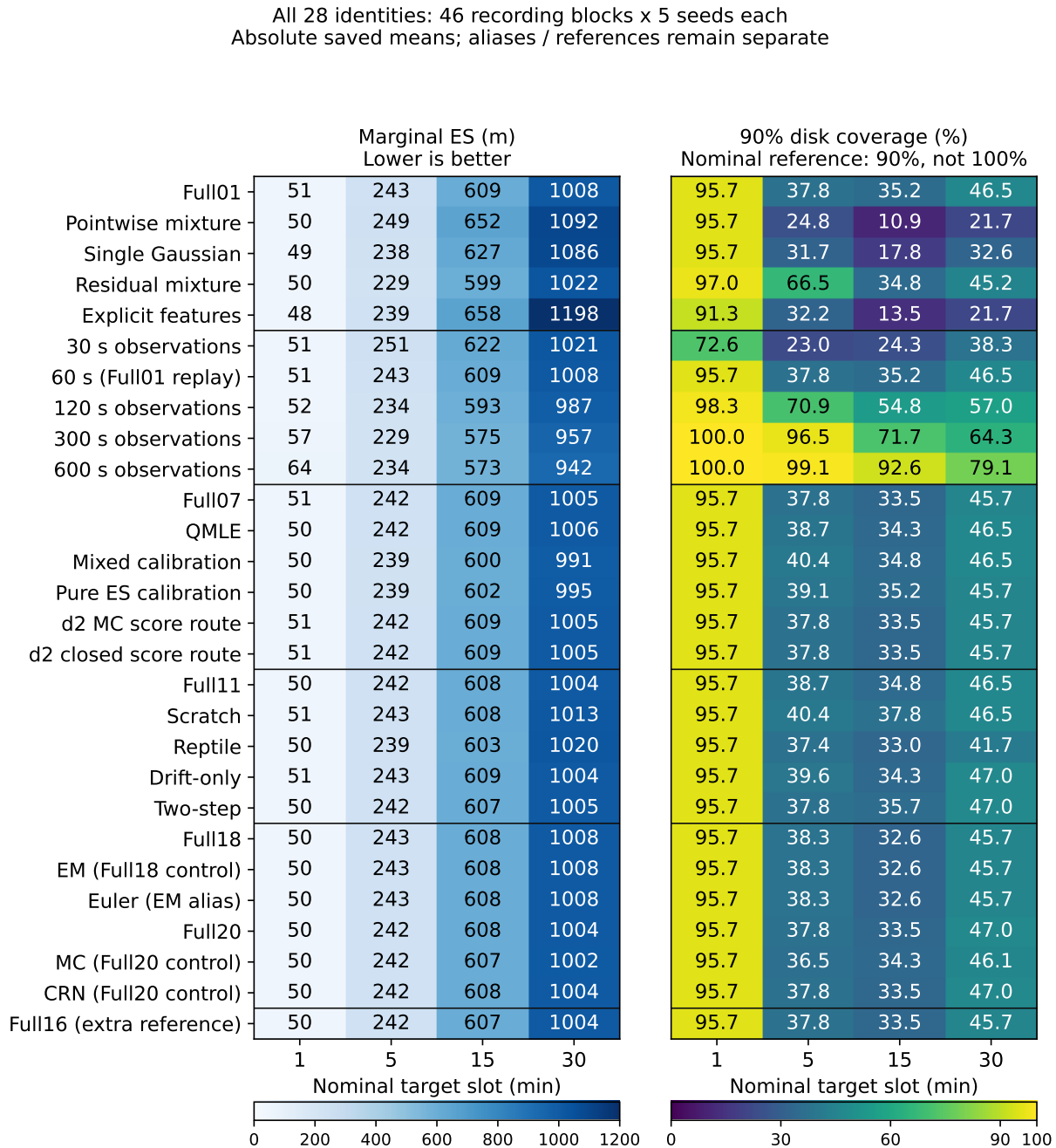
图 4: 全部 28 个主组保存配置在四个名义目标时域的概览; 没有新增中间时刻预测。左: 边际 ES (米), 越低越好。右: 名义 90% 预测圆的实际覆盖率 (%); 校准参考是 90% 而不是 100%, 本图不显示区域大小。每格平均同一 46 块、五个种子。概览 ES 舍入到整数米, 覆盖率保留一位小数; 完整精度和全部角色保留于保存投影及表 49。行按登记家族而非性能排序; 别名与不同 Full 对照不合并, 舍入相似不证明等价。这是描述展示, 不是新增逐时域检验或最终资格。
