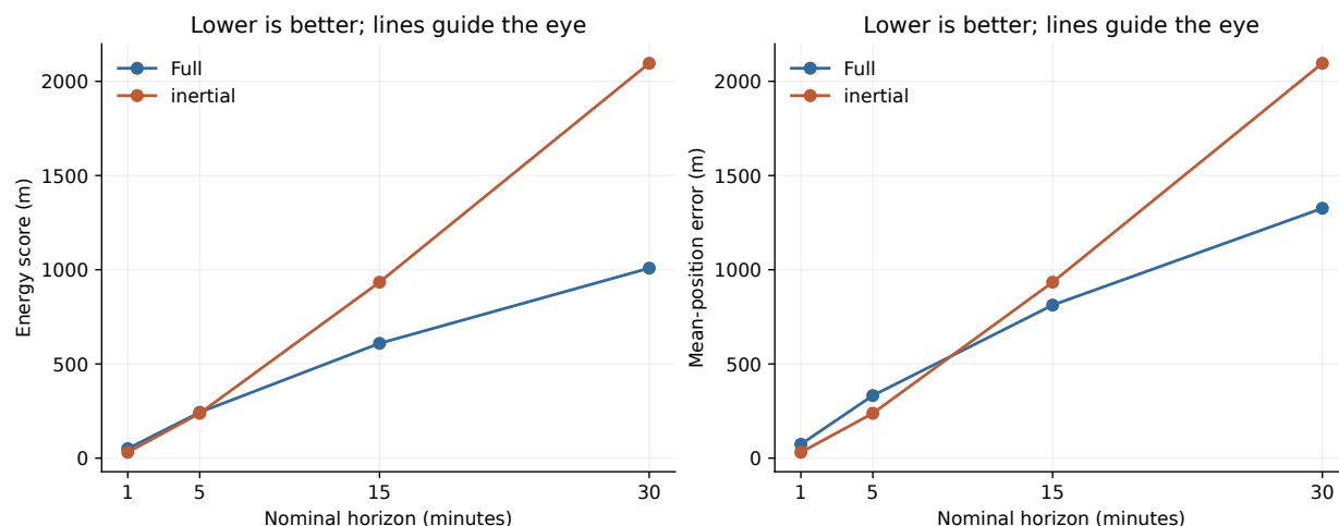
图 3: Full 与确定性惯性四时域对照：左为 ES，右为预测均值误差，采用原等块 / 等种子汇总。连线只引导阅读，不代表连续插值或精确交叉时刻。
