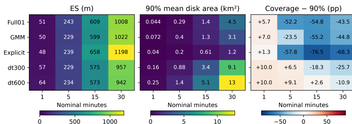
图 4: 按角色选择的概览：参考、残差混合、显式表示及长观测间隔。行按科学角色固定，不按已见性能排名。ES 与面积使用全 28 身份的范围；覆盖偏差为观测减 90% 的百分点，带符号数值使方向不依赖配色。
