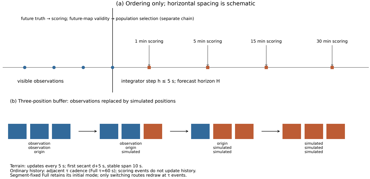
图 1: 可见观测与模拟历史。 \tau 为观测 / 模型节拍， h 为积分步长， H 为预测时长。地形三位置缓冲按 5 秒事件更新，全为模拟点后割线跨度 10 秒；普通 Full 另有 \tau = 60 秒节拍。未来观测只进入评分；评分事件本身不更新历史。图内固定英文符号与本文定义对应。
