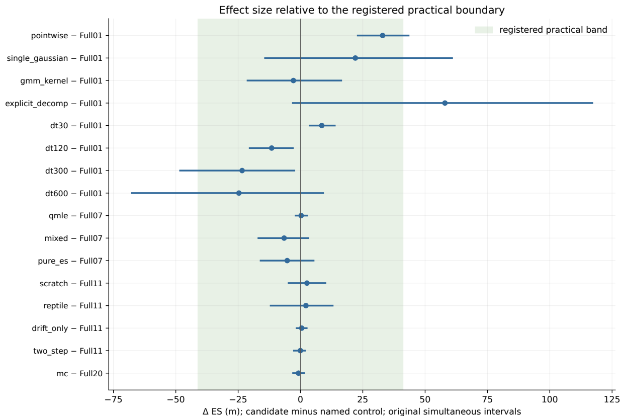
图 5: 原配对 ES 效应与同时区间，保留具名候选 / 对照和 \pm 41.10 米实际带。微小实现一致性差值在补充材料用独立尺度显示，不删除、不解释为科学大效果。区间位置与程序资格分别判断。
