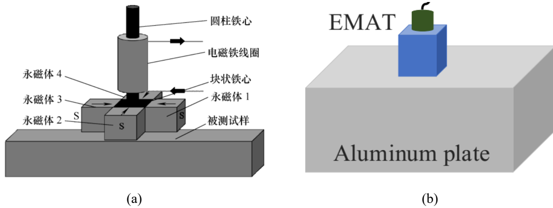
图 1-5 EMAT 换能器的两种典型磁场优化设计。(a) 磁力可控电磁超声换能器——通过永磁体与电磁铁组合控制磁场强度，实现磁场总体的增强与削弱，解决粗糙表面上的声速测量偏差；(b) 基于电磁超声体波的铝板缺陷检测换能器——采用洛伦兹力体波激励机制，在非铁磁材料（铝）中实现无耦合剂测厚。
