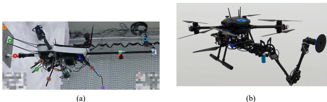
图 1-6 全驱动平台在接触式 NDT 中的两种典型实现。(a) 利用 Voliro 全矢量推力六旋翼——通过可倾转旋翼实现位置-姿态动力学解耦，在倾斜和悬垂表面上完成干耦合超声 B 扫描，法向力维持在 20 N；(b) 基于倾转旋翼平台的半自主 NDT 框架——双重阻抗控制（机械臂端精细力控 + 机体端姿态稳定）解耦运行，动态吸收接触冲击扰动。
