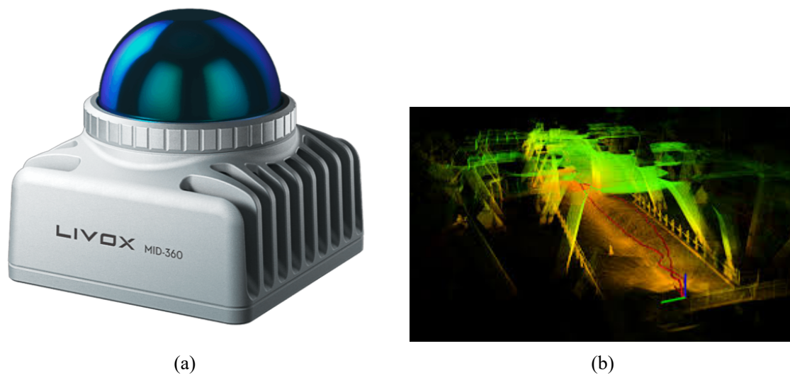
图 3-3 (a) Livox MID-360 固态激光雷达；(b) FAST-LIO2 紧耦合里程计定位效果
