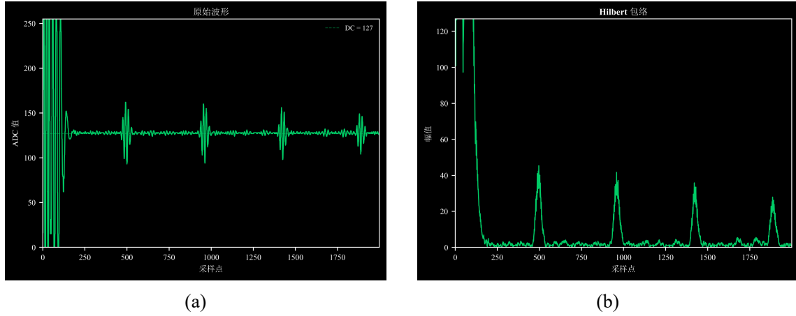
图 2-1 接触状态下 EMAT 回波波形。原始波形呈现周期性的多次底面反射回波序列；Hilbert 包络显示幅值沿传播时间呈稳定指数衰减，相邻回波时间间隔 \Delta t 对应单程渡越时间。
