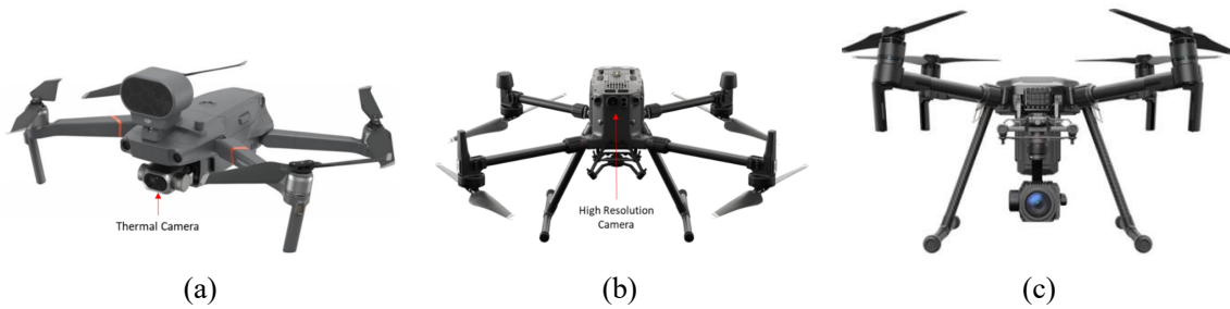
图 1-2 无人机视觉巡检技术的三个代表性方向。(a) Omar 和 Nehdi [7] 利用无人机搭载红外热像仪对混凝土桥面板进行非接触脱粘检测，通过 k -means 聚类分割热图生成损伤状态图；(b) Feroz 和 Abu Dabous [8] 对 65 篇无人机桥梁检测文献的系统综述，涵盖可见光、红外热成像、LiDAR 和 NDT 传感器等多种模态；(c) Memari 等人 [9] 综述了无人机与深度学习技术在风电叶片缺陷检测中的融合应用，覆盖裂纹、侵蚀和涂层异常等损伤类型。
