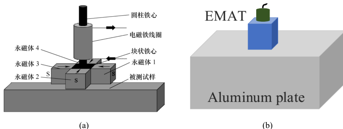
图 1-5 EMAT 换能器的两种典型磁场优化设计。(a) 磁力可控电磁超声换能器——通过永磁体与电磁铁组合控制磁场强度，实现磁场总体的增强与削弱，解决粗糙表面上的声速测量偏差；(b) 基于电磁超声体波的铝板缺陷检测换能器——采用洛伦兹力体波激励机制，在非铁磁材料（铝）中实现无耦合剂测厚。
