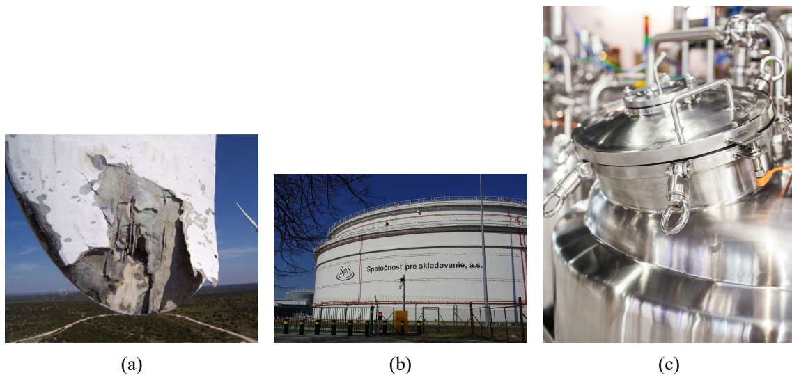
图 1-1 无人机无损检测面向的典型复杂工业结构。(a) 风力发电机叶片——大型复合材料结构，长期暴露于风沙、雨水和紫外线，表面裂纹、分层和前沿侵蚀是常见损伤模式；(b) 储罐壁板——大型圆柱形钢制容器，受内压与腐蚀介质作用，壁厚减薄和点蚀是检测重点；(c) 压力容器——不锈钢工业容器，焊缝退化和应力腐蚀裂纹是主要安全隐患。三类结构均位于高空或受限空间，构成无人机接触式 NDT 的核心应用场景。
