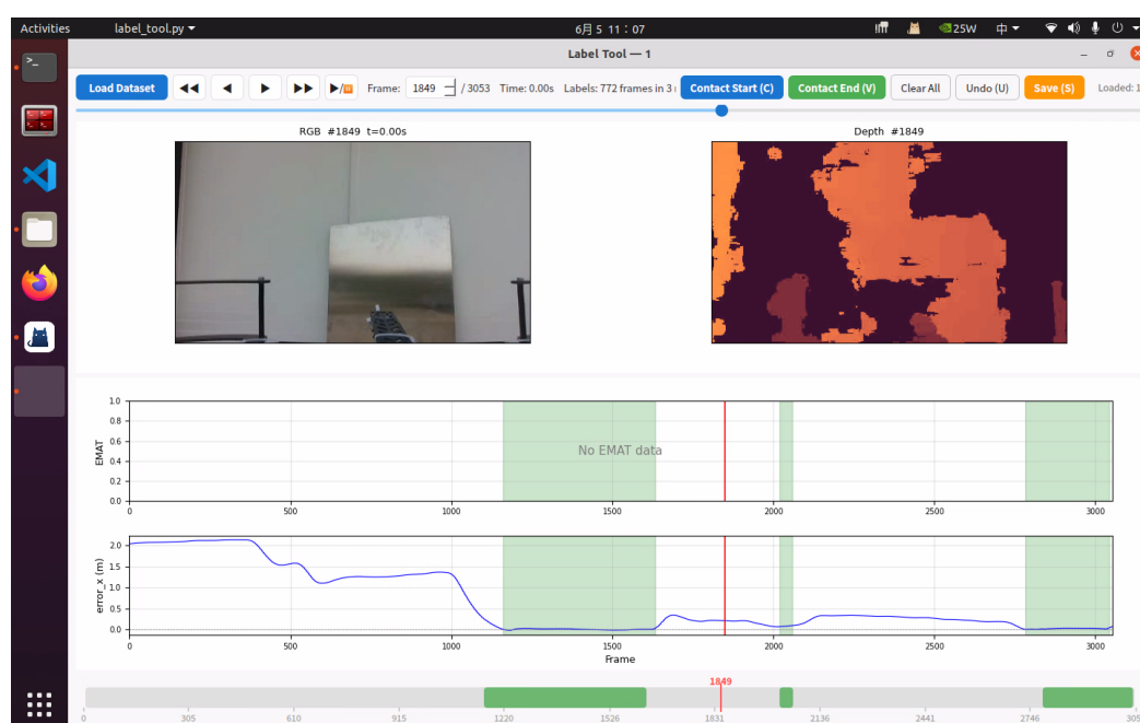
图 3-6 PyQt5 接触标签标注工具界面
