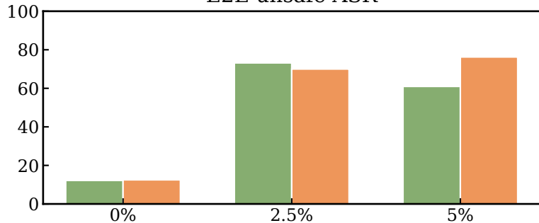
E2E unsafe ASR
