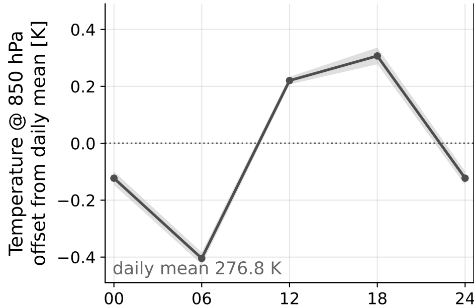
ERA5 1955
