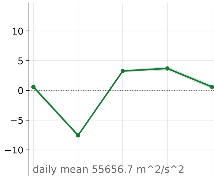
ERA5 2023
