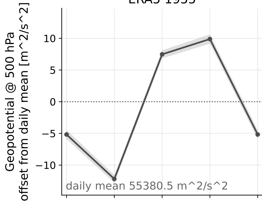
ERA5 1955
