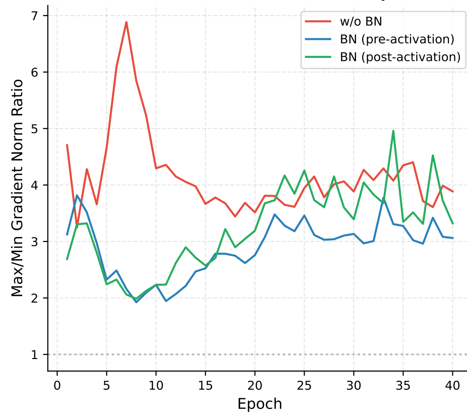
(d) Gradient Norm Ratio Across Layers
