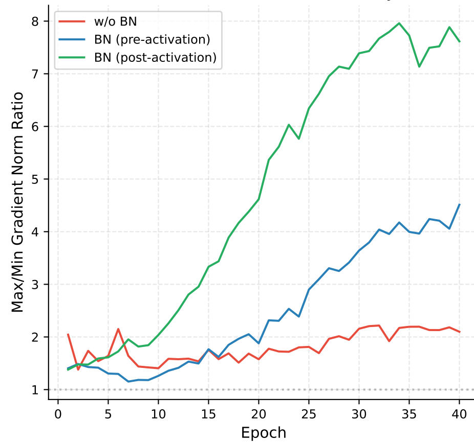
(d) Gradient Norm Ratio Across Layers
