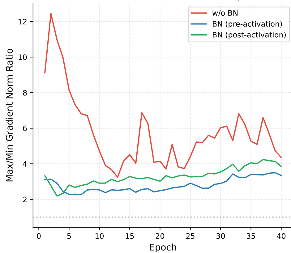
(d) Gradient Norm Ratio Across Layers
