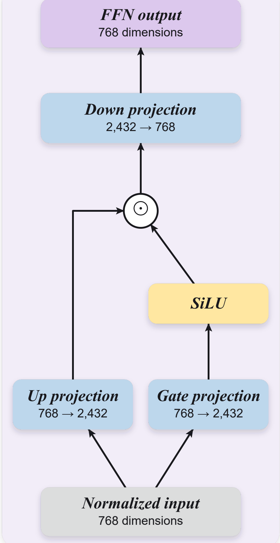
(d) SwiGLU FFN
