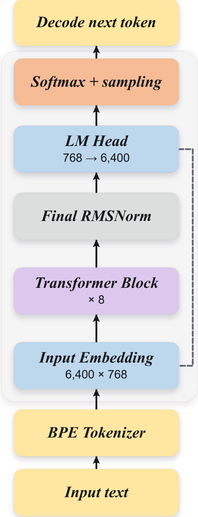
(a) Autoregressive LM
