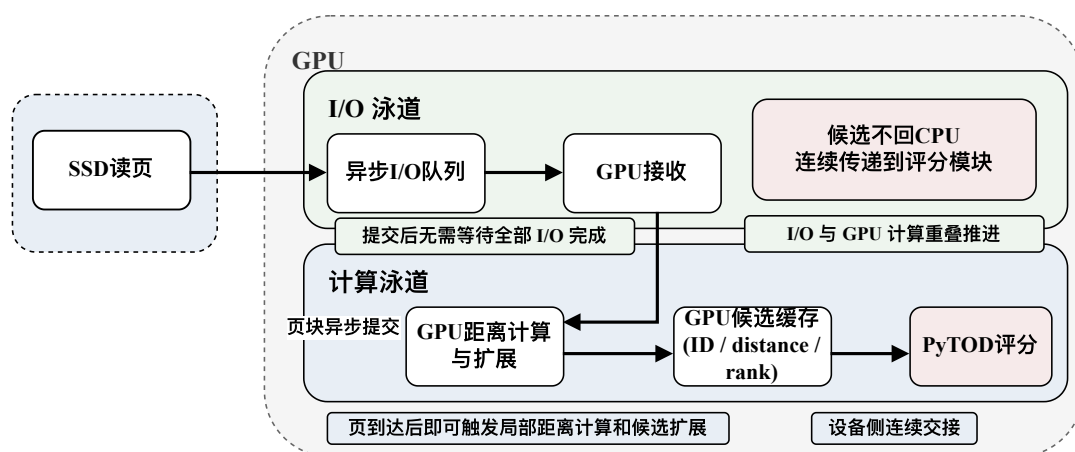
图 4-3 外存 ANNS 异步 I/O—计算流水线与本文候选召回前端接入方式（根据文献 [7] 和本文系统实现整理）
