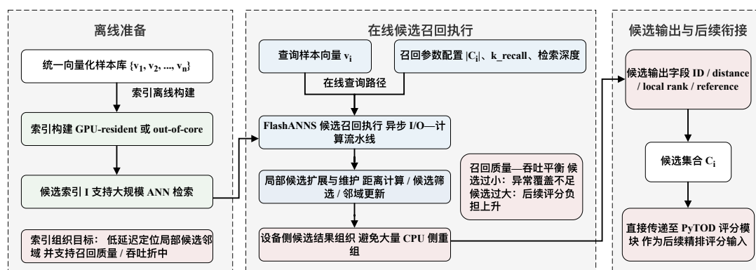
图 3-4 FlashANNS 候选召回执行流程图
