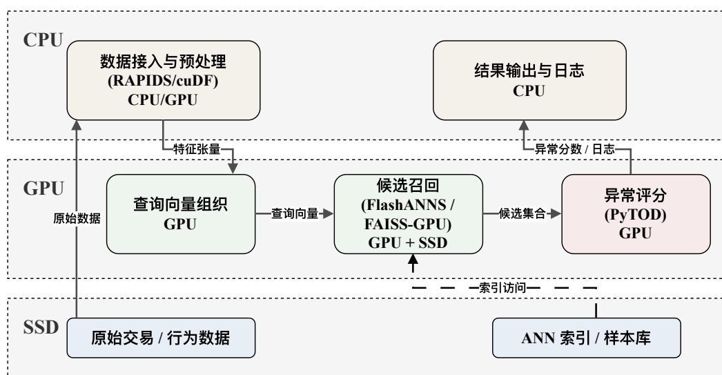
图 4-1 单卡异常检测系统总体架构图
