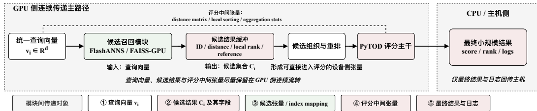
图 3-5 模块间中间结果传递示意图
