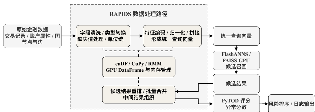
图 2-4 RAPIDS 在本文系统中的数据处理位置
