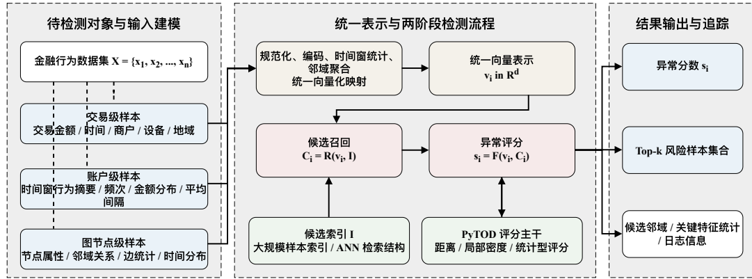
图 3-1 金融异常检测任务建模图
