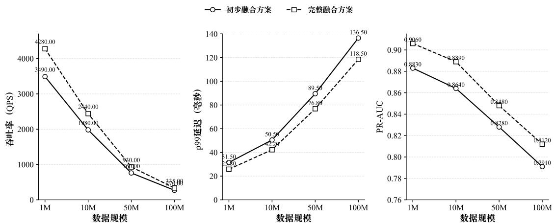
图 6-7 不同规模下系统表现趋势
