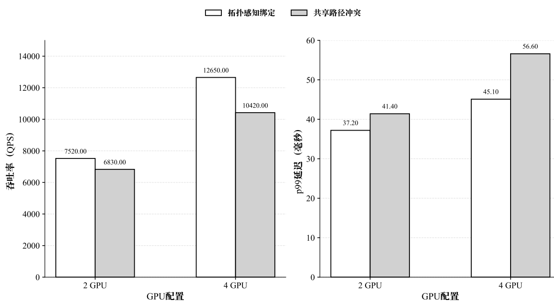
图 5-6 I/O 通道配置对扩展性的影响
