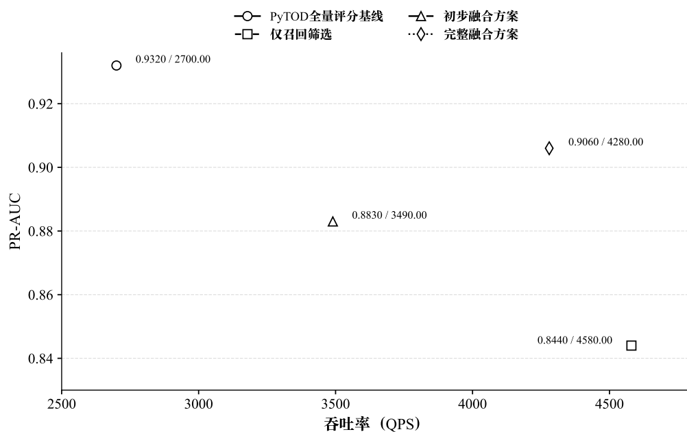
图 6-6 FlashTOD 效果与性能折中
